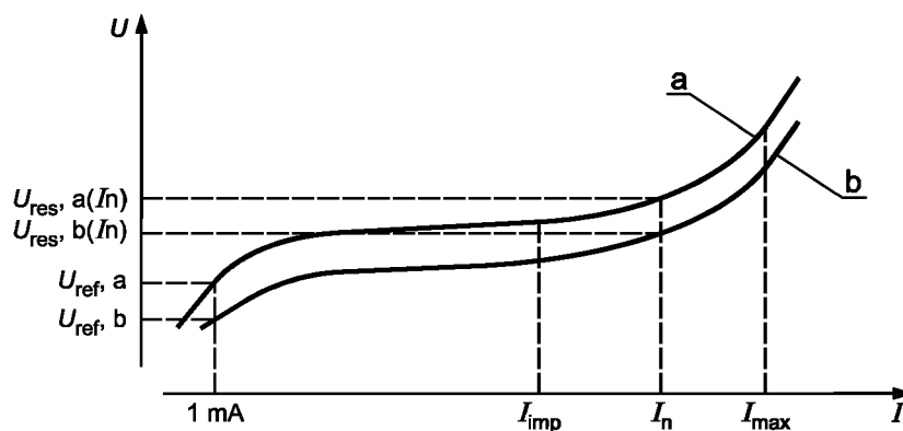
Рисунок E.14 — Два варистора ZnO с одинаковым номинальным разрядным током
