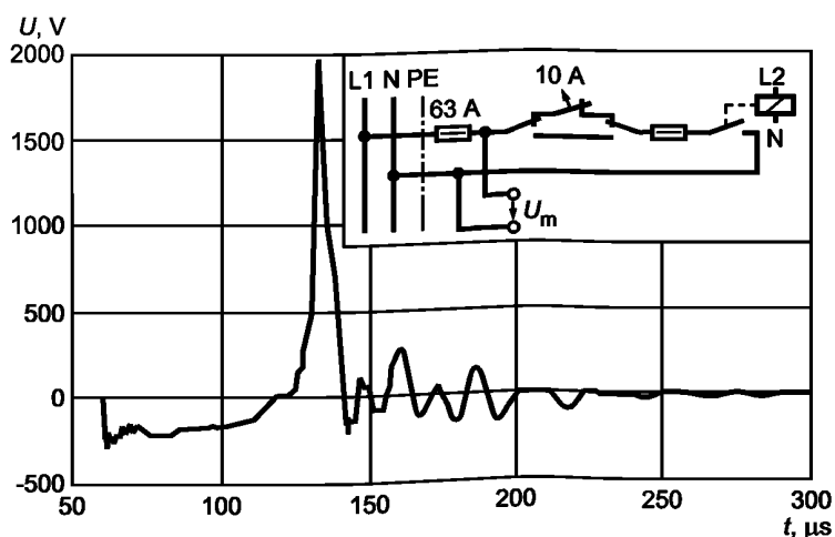
Рисунок 21 — Импульсные коммутационные перенапряжения при срабатывании миниатюрного предохранителя
