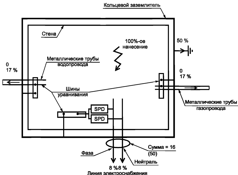
Рисунок 24 — Пример проникновения тока молнии во внешние коммуникации (система ТТ)
