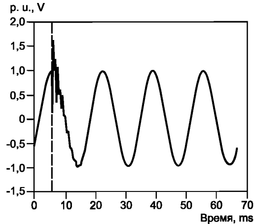
Рисунок В.3 — Типовое перенапряжение, возникающее при подключении конденсаторной батареи
