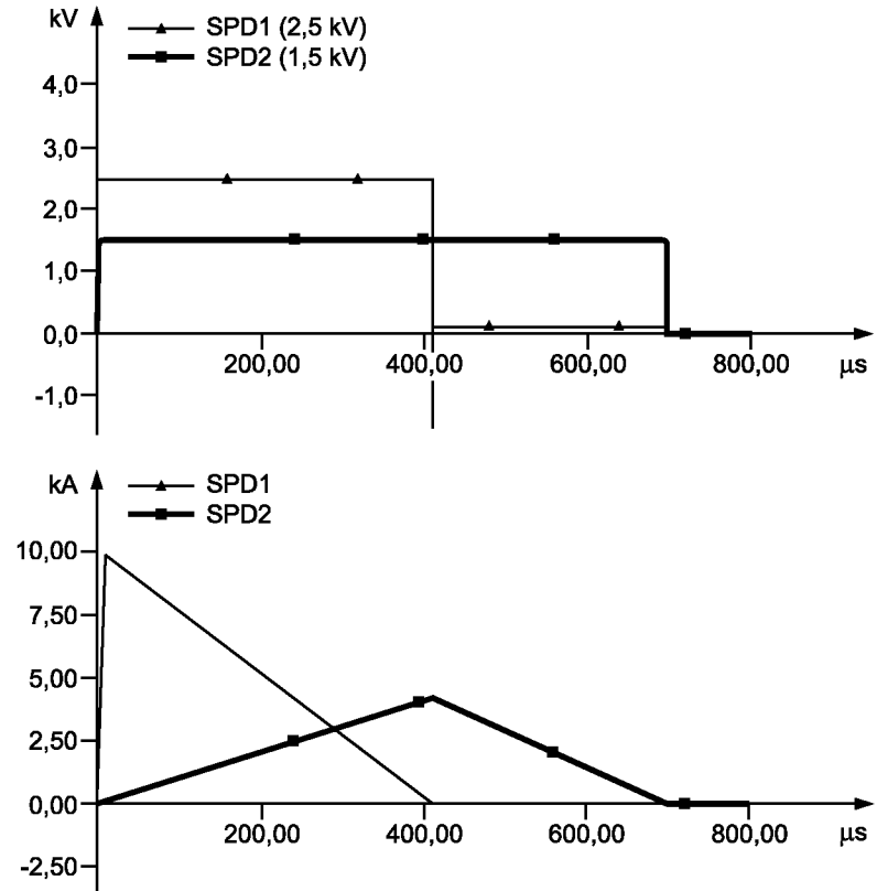
Рисунок Е.8 — Расчетные напряжения и ток УЗИП для импульса тока 10/350 мкс, введенного в узле 1
