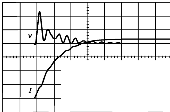
I Входной ток NID 50 А/div: di/dt = 75 А/мкс V Напряжение между телефонным портом и защитным проводником (PE) 2 кВ/дел: максимум 4,3 кВ. Горизонтальная развертка: 2 мкс/дел
