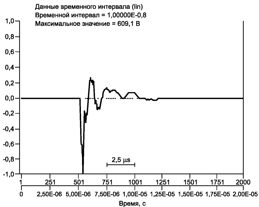
Рисунок 15 — Пример высокочастотного импульса коммутационного перенапряжения
