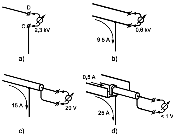
Рисунок F.3 — Измерение напряжения в диспетчерской на кабеле, замкнутом на первичной стороне трансформатора. Токи обычного вида для различных параллельных заземляющих проводников между точками А и С.
