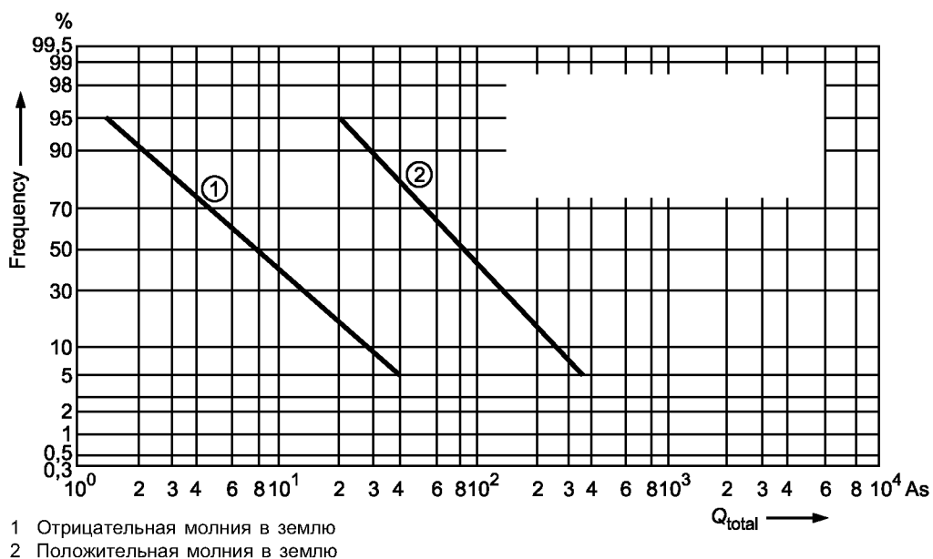
Рисунок А.2 — Частотное распределение полного заряда молнии Q_{total}
