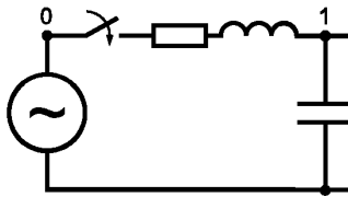
Рисунок 13 — Генерация перенапряжения при коммутации цепи RLC
