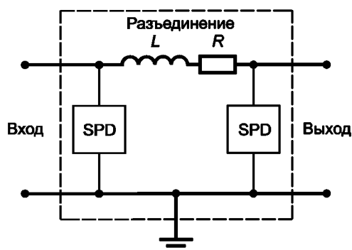
Рисунок Е.19 — Принцип координации для вида IV
