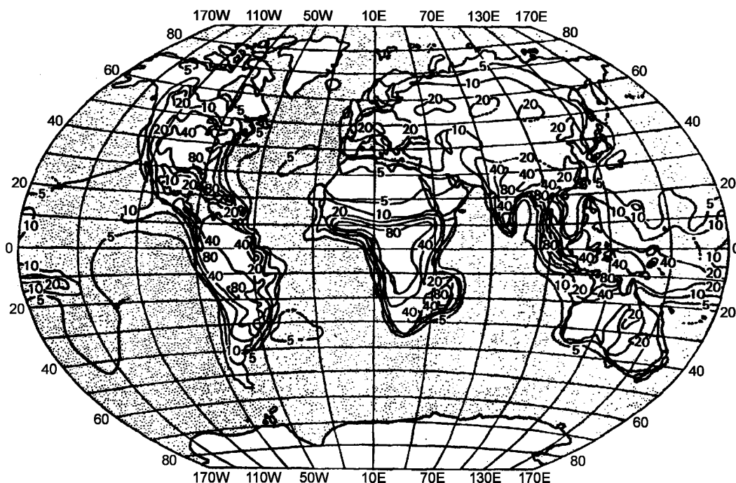
Рисунок 5 — Карта интенсивности гроз 1)
