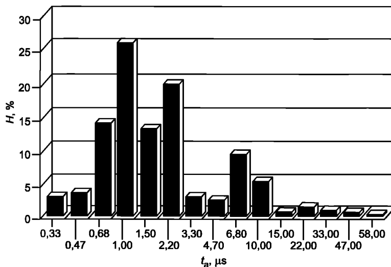
Рисунок 17 — Распределение импульсных коммутационных перенапряжений по времени
