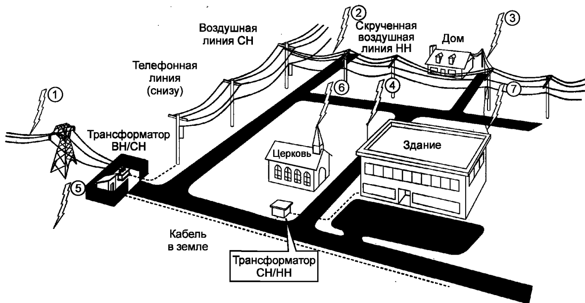
Рисунок 1 — Примеры механизмов воздействия при ударе молнии
