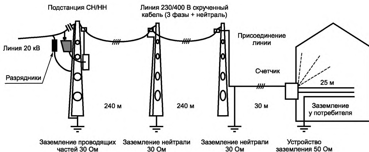
Рисунок 11 — Модель системы электроснабжения
