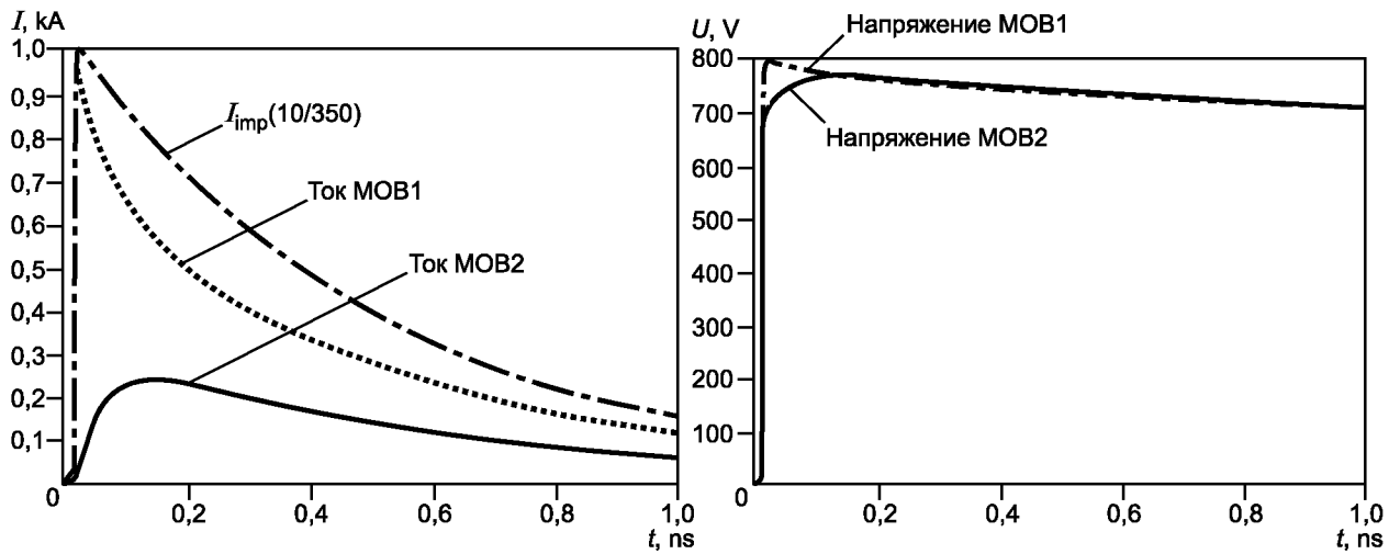
Рисунок Е.3 — Зависимости тока и напряжения от времени для двух ограничивающих напряжение УЗИП
