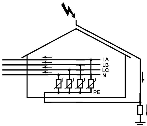
Рисунок 7 — Пример резистивной связи с системой молниезащиты
