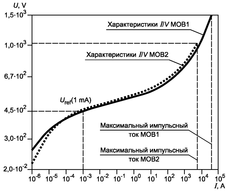
Рисунок Е.2 — Сравнение вольтамперных характеристик двух MOV
