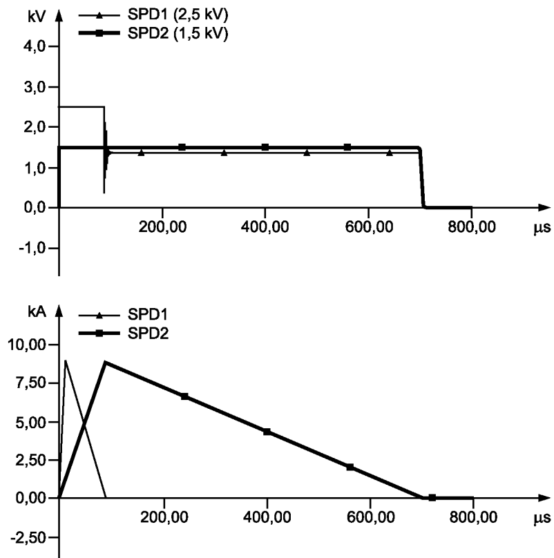
Рисунок Е.7 — Расчетные напряжения и ток УЗИП для импульса тока 10/350 мкс, введенного в узле 2
