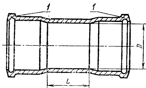
1 — раструбы типа II по ГОСТ 6942.2—80
