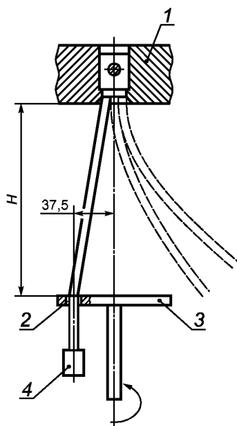
1 — узел фиксации; 2 — гильза; 3 — диск; 4 — груз
