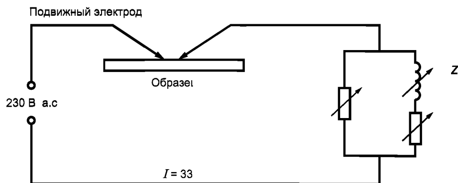
Рисунок М.2 — Схема испытания на воспламеняемость электрической дугой
