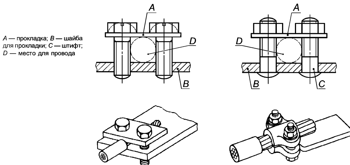
Рисунок D.3 — Штифтовой вывод
