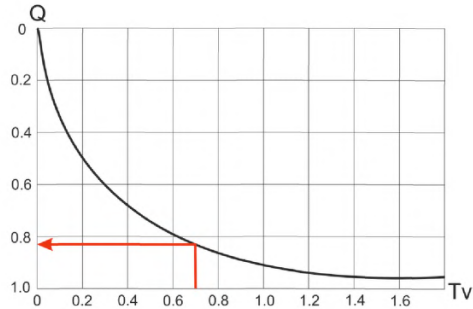
Рисунок 8 – Зависимость степени консолидации в вертикальном направлении Q от фактора времени T_v
