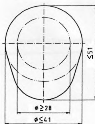
Рисунок 2 – Профиль жерди
