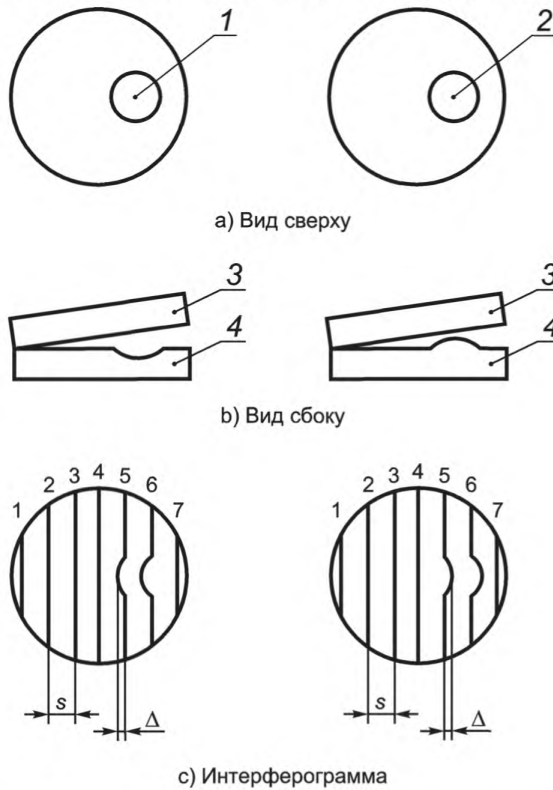
1 — вогнутость; 2 — выпуклость; 3 — опорная поверхность; 4 — измеряемая поверхность; 5 — расстояние между полосами при наилучшей аппроксимации интерференционной картины; \Delta — максимальное отклонение от наилучшей аппроксимации интерференционной картины
