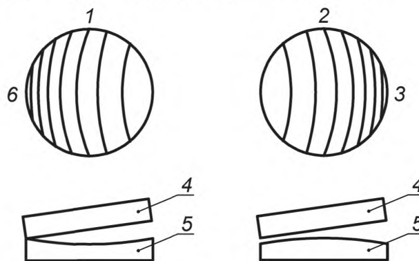
1 — вогнутая сфера; 2 — выпуклая сфера; 3 — утолщенная часть клина; 4 — опорная пластина; 5 — измеряемая поверхность; 6 — суженная часть клина
