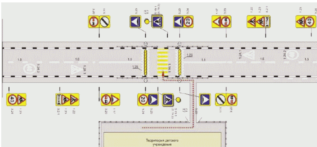
Рисунок Д.7 - Комплексное обустройство ТСОДД нерегулируемого пешеходного перехода вблизи детских учреждений
