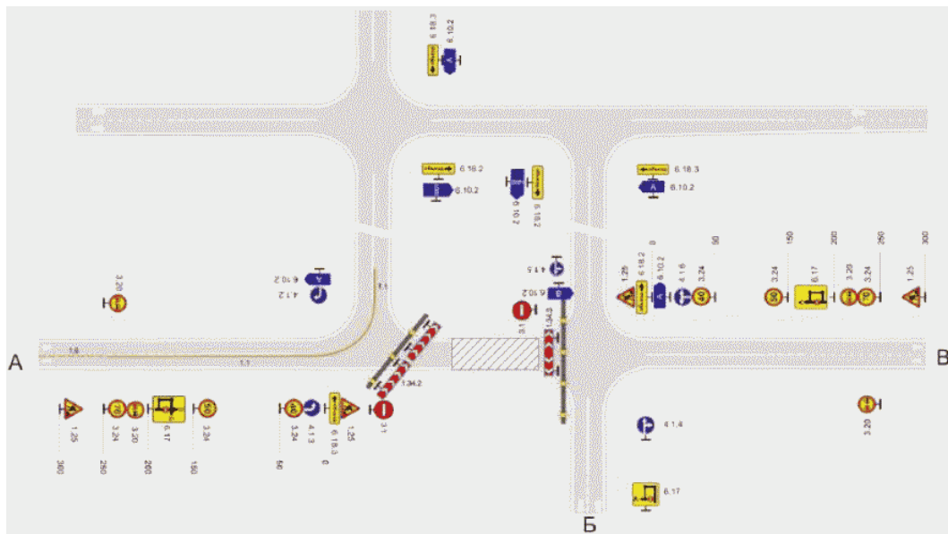
Рисунок Д.23 - Общая схема расстановки временных дорожных знаков при производстве долгосрочных дорожных работ на участке дороги с полным закрытием проезжей части и организацией объезда
