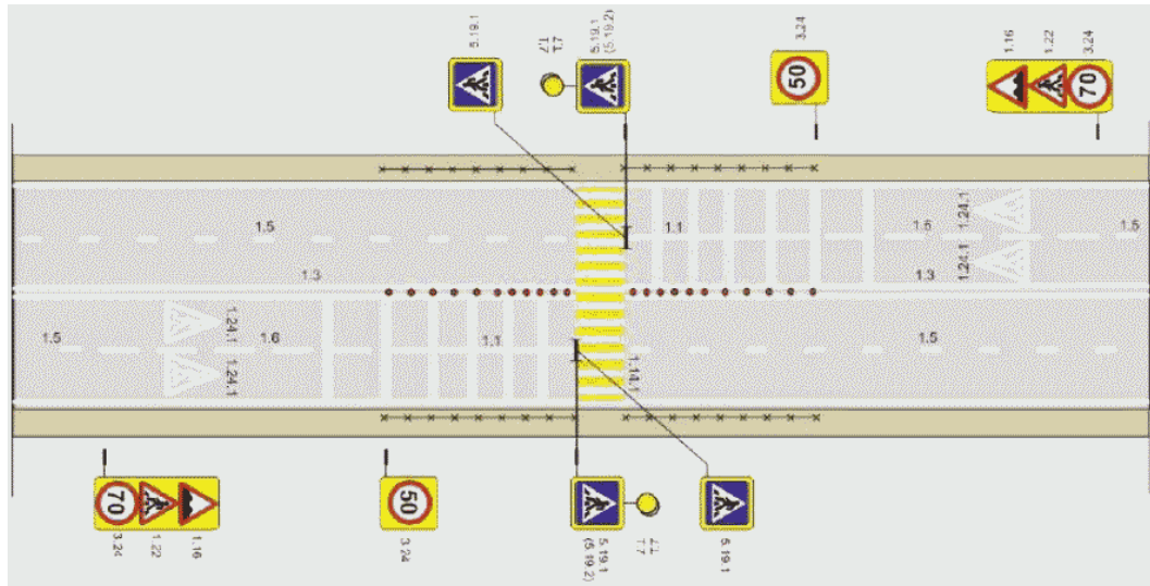
Рисунок Д.10 - Установка ТСОДД в зоне регулируемого пешеходного перехода на участке дороги с четырьмя полосами и более с разделительной полосой
