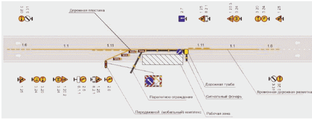
Рисунок Д.24 - Размещение ТСОДД при производстве долгосрочных работ на проезжей части дороги с двумя полосами
