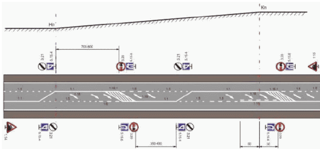
Рисунок Д.18 - Организация движения и установка знаков на подъемах и спусках дорог с тремя полосами: а - на спусках и подъемах длиной менее 1200 м; б - на затяжных спусках и подъемах длиной 1200 м и более (Hн - начало подъема; Кп - конец подъема)
