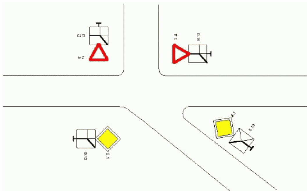
Рисунок Д.1 - Размещение знаков приоритета на главной дороге перед перекрестком, на котором главная дорога изменяет направление
