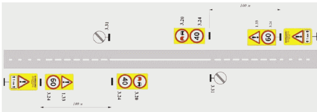
Рисунок Д.14 - Применение ТСОДД на прямых горизонтальных
