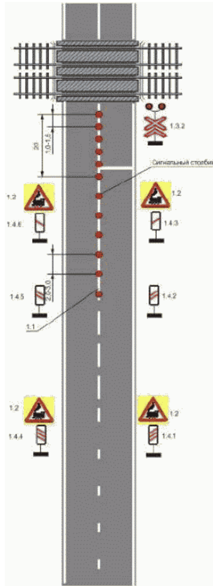
Рисунок Д.13 - Размещение сигнальных столбиков на подходе к железнодорожному переезду
