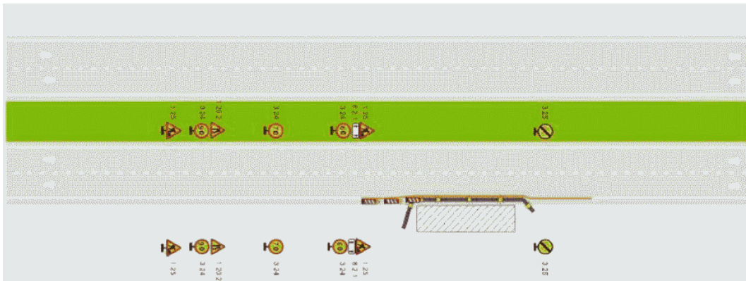
Рисунок Д.28 - Размещение ТСОДД при производстве долгосрочных работ на обочине дороги с четырьмя полосами
