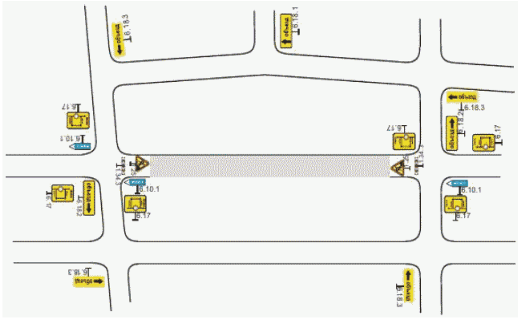
Рисунок Д.22 - Общая схема расстановки временных дорожных знаков 6.17 и 6.18.1 - 6.18.3 на УДС при производстве долгосрочных дорожных работ на улице с полным закрытием проезжей части и организацией объезда
