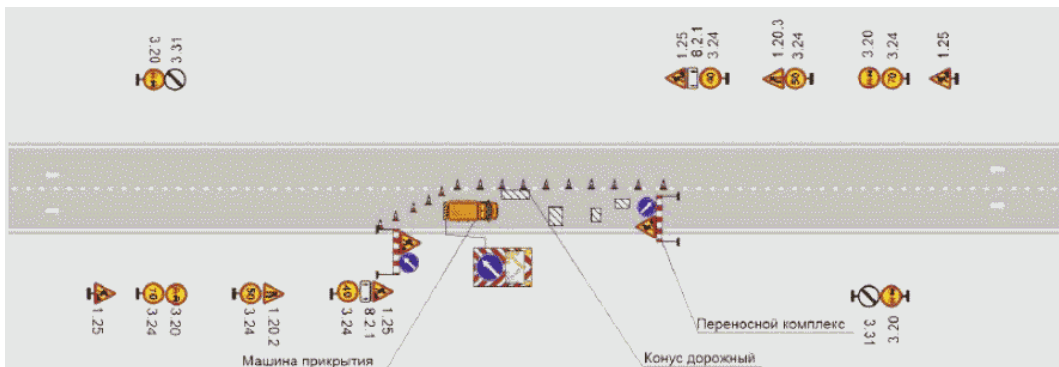
Рисунок Д.26 - Размещение ТСОДД при производстве краткосрочных работ на проезжей части дороги с двумя полосами
