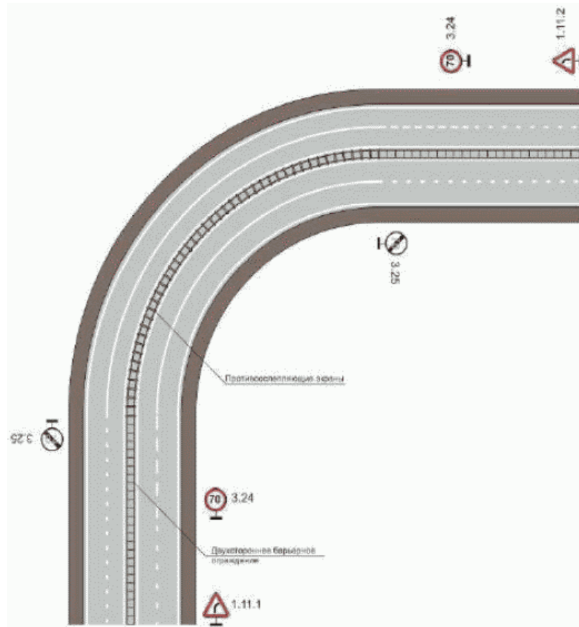
Рисунок Д.15 - Установка элементов обустройства дороги на крутых (опасных) поворотах: а - дороги с тремя полосами; б - дорога с четырьмя полосами
