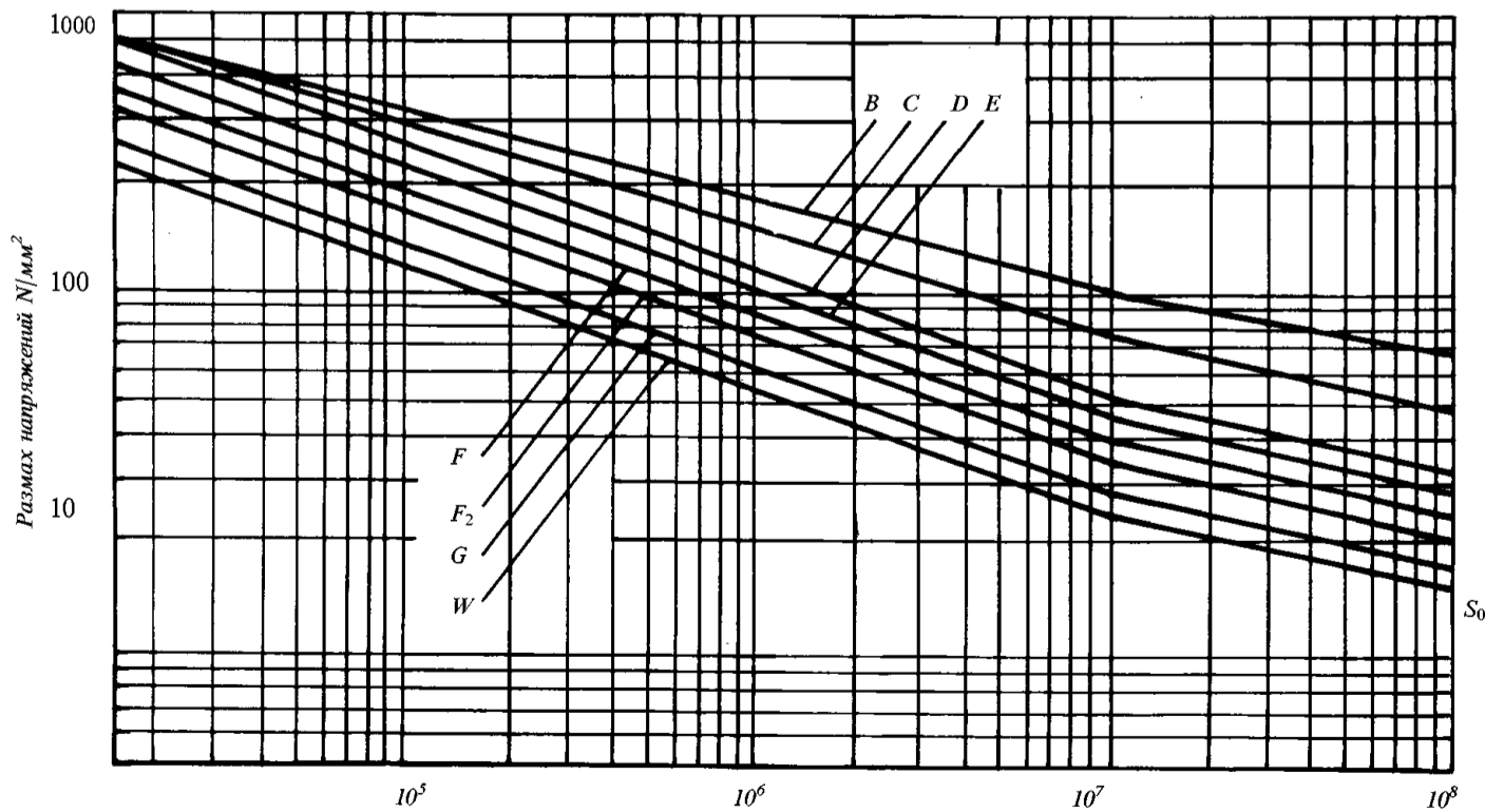
Рис. 2.4.4.8-1 Кривые усталости
