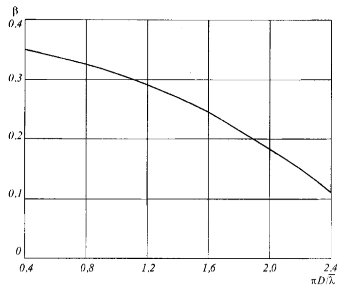
Рис. 3.3.2.1.8.2 Зависимость коэффициента \beta от \pi D / \lambda
