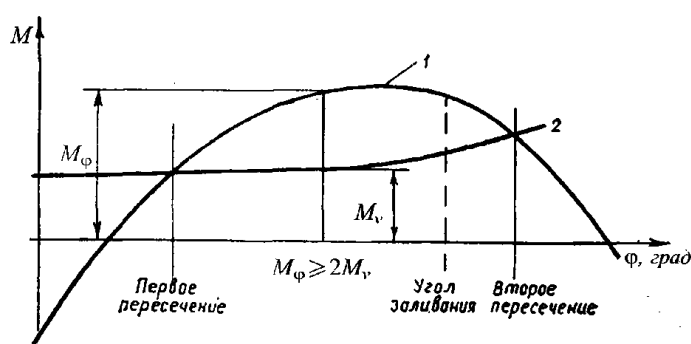
Рис. 2.6.2.1.4 Кривые восстанавливающего момента (1) и ветрового кренящего момента (2)
