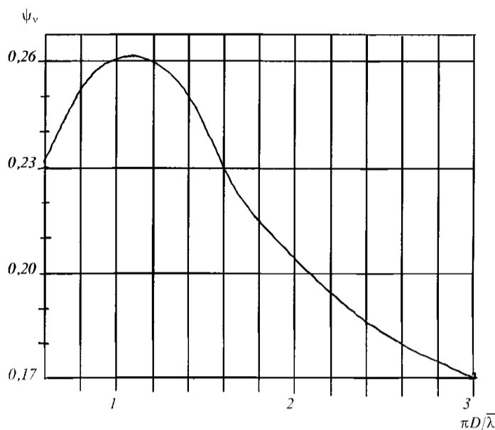
Рис. 3.3.2.1.7 Значение параметра \psi_v дополнительного опрокидывающего момента
