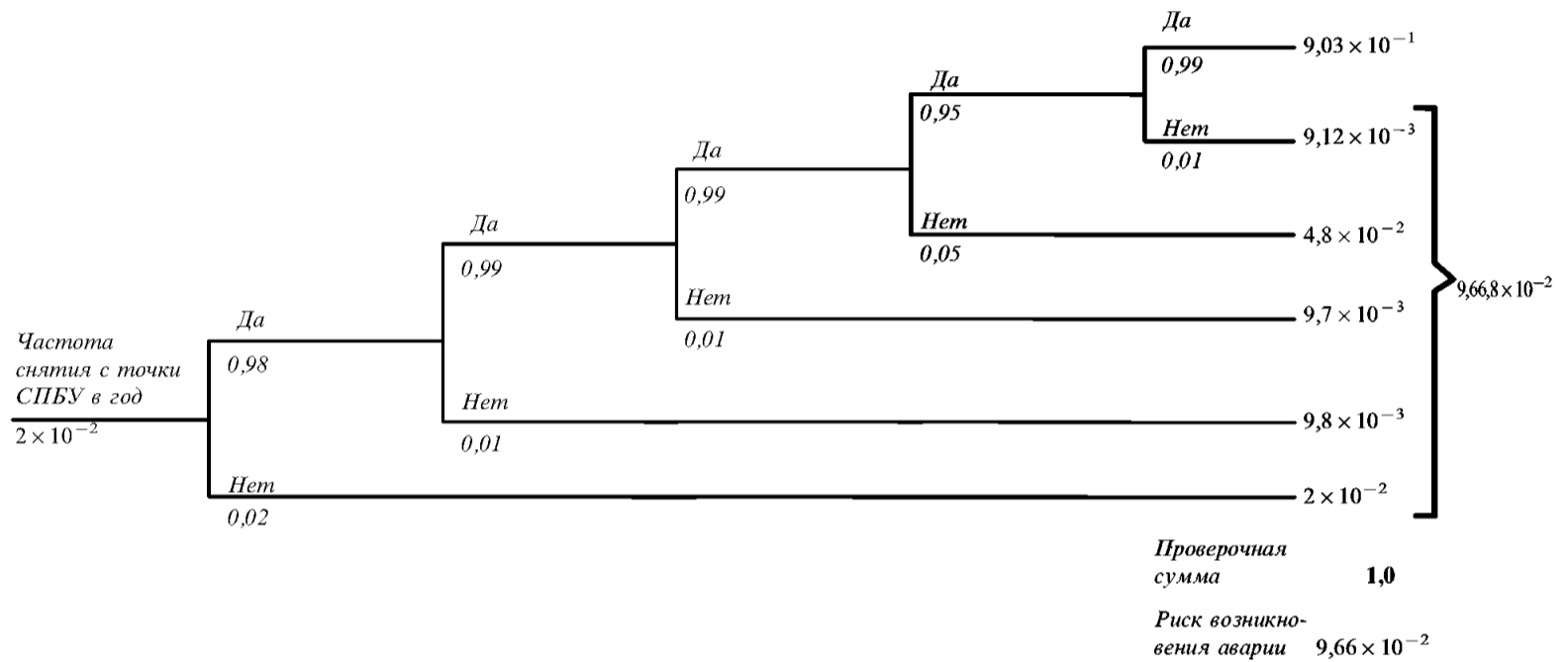
Дерево событий при транспортировках СПБУ и ППБУ
