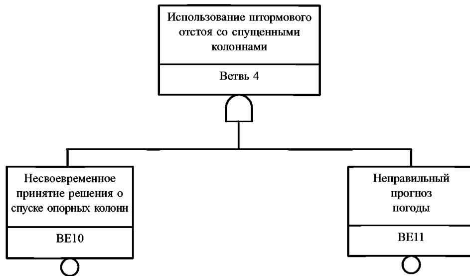
Продолжение построения дерева ошибок и неполадок
