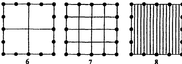
Рис. П.Е.1. Сложные заземлители
