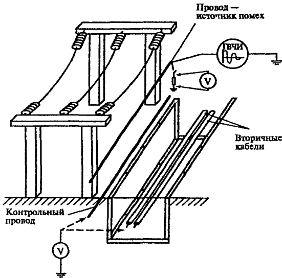
Рис. 6. Схема имитации излучаемых помех
