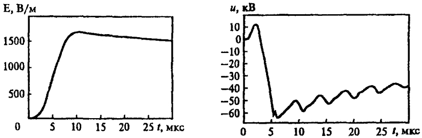
Рис. П.Е.3. Расчет напряженности электрического поля молнии и напряжения наводки на воздушной линии по программе
