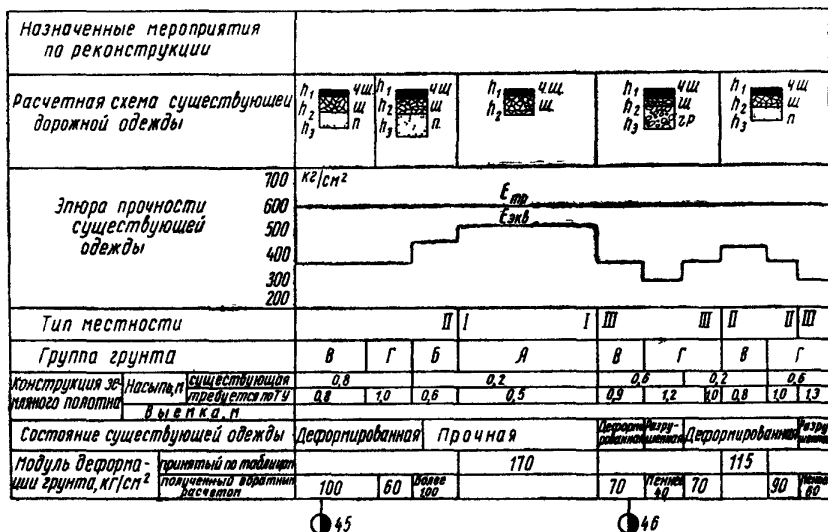
Рис 7 Эпюра прочности дорожной одежды
