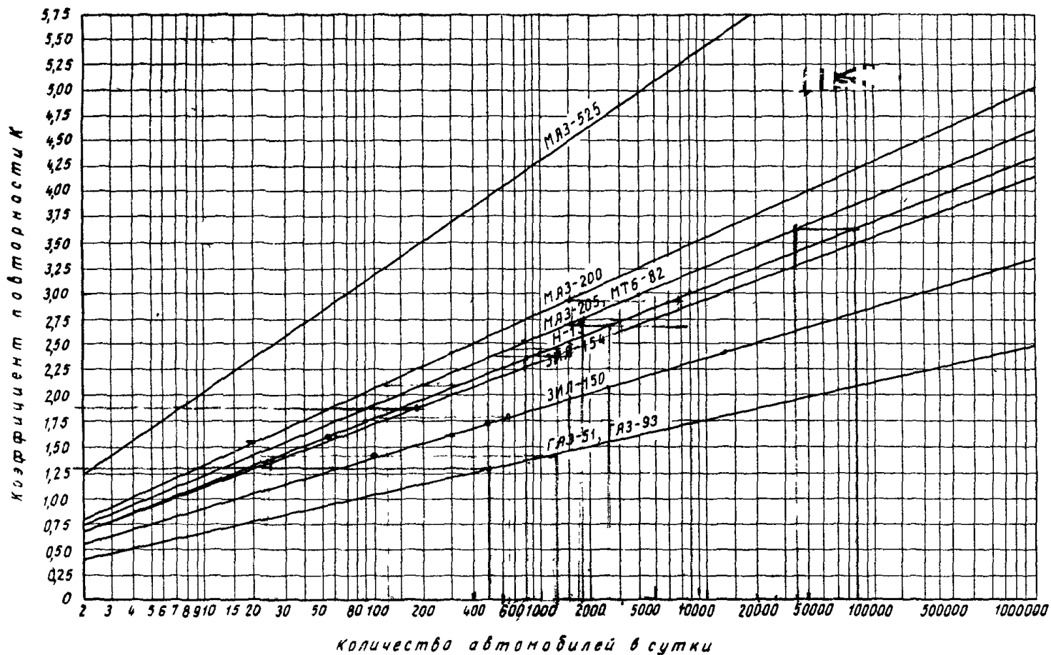
Рис 2. График для приведения интенсивности движения к расчетной H-13
