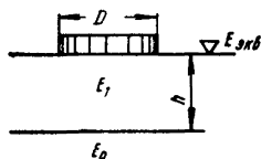
Рис. 4 Расчетная схема двухслойной системы
