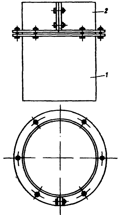
Рис 10. Форма со съемной надставкой:
