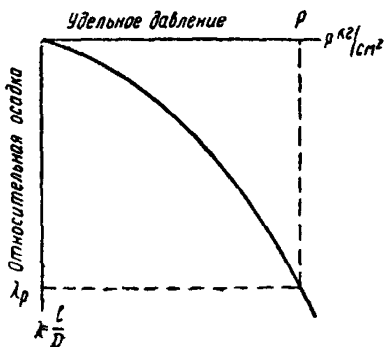
Рис. 9 Кривая зависимости относительной осадки от удельного давления
