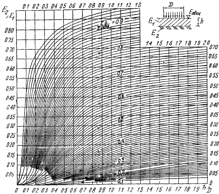
Рис. I. Номограмма для определения модуля упругости E_1 верхнего слоя двухслойной системы
