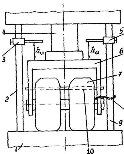
Рис.3.Схема тарировки колеса для установки УДН-НБ:
