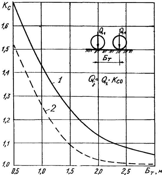
Рис. I. Зависимость коэффициента влияния смежной оси ( K_c ) от базы тележки ( B_t ), м:
