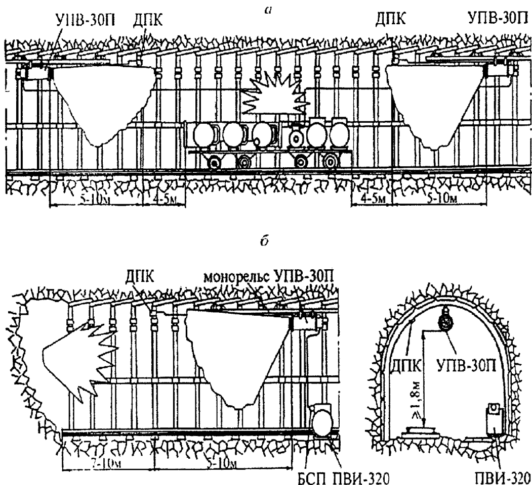
Рис. 1. Схемы установки СЛВА в горных выработках:
