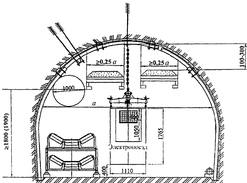
Рис. 6. Схема установки сланцевых заслонов в выработке сечением не менее 19,2 м 2 , закрепленной металлической арочной крепью из специального профиля и оборудованной ленточным конвейером и монорельсовым транспортом
