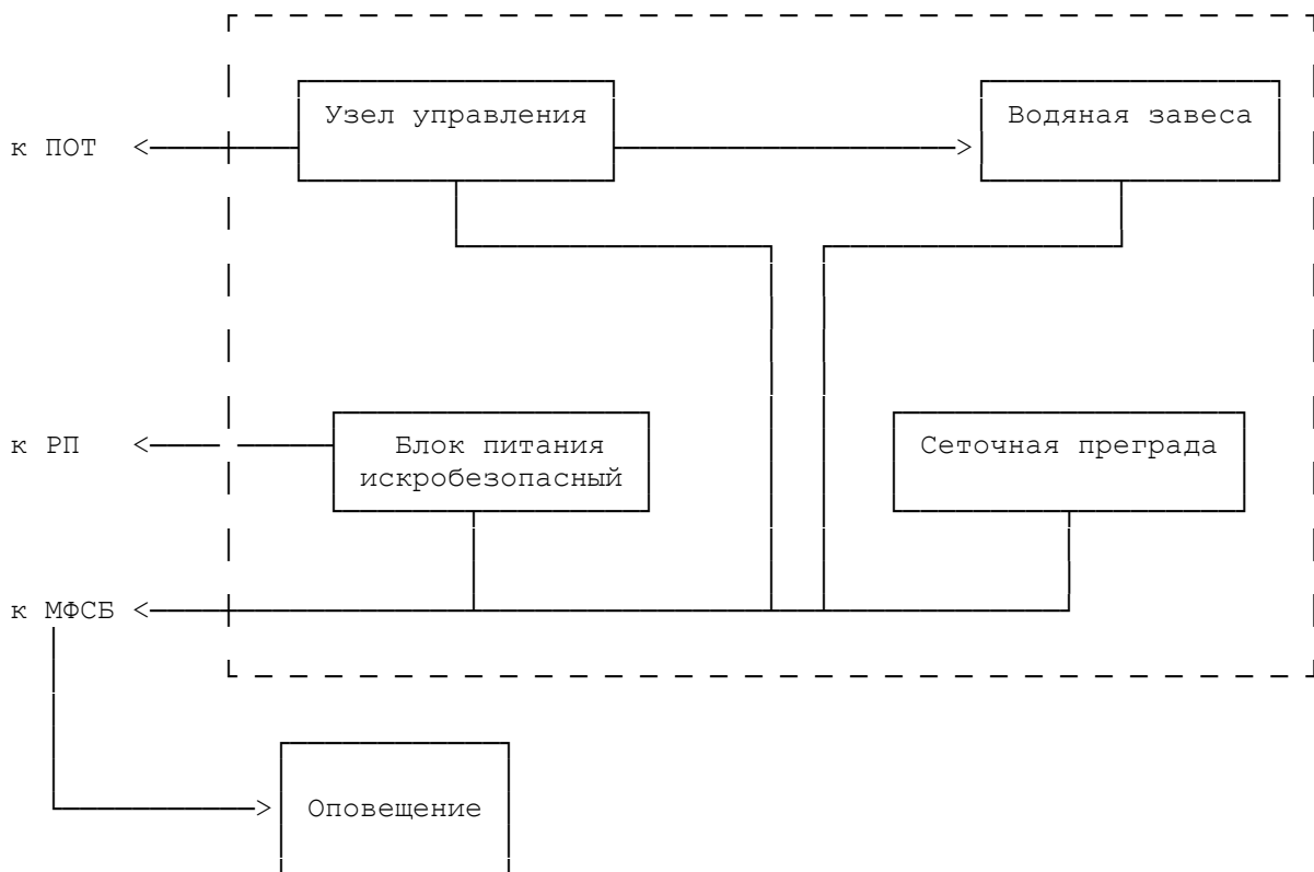
Рис. 1. Блок-схема подключения АВЗ:
