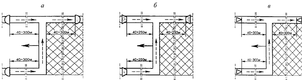
Рис. 5. Схемы установки заслонов от сопряжения с очистной выработкой в конвейерной выработке и в вентиляционной выработке, по которой отводится вентиляционная струя при прямоточных с подсыжением схемах проветривания
