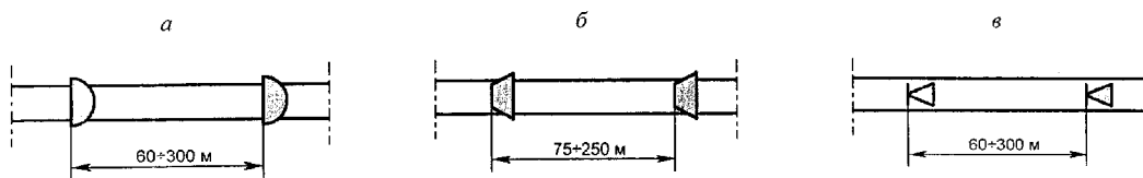
Рис. 7. Схемы установки заслонов в выработках, оборудованных ленточными конвейерами
