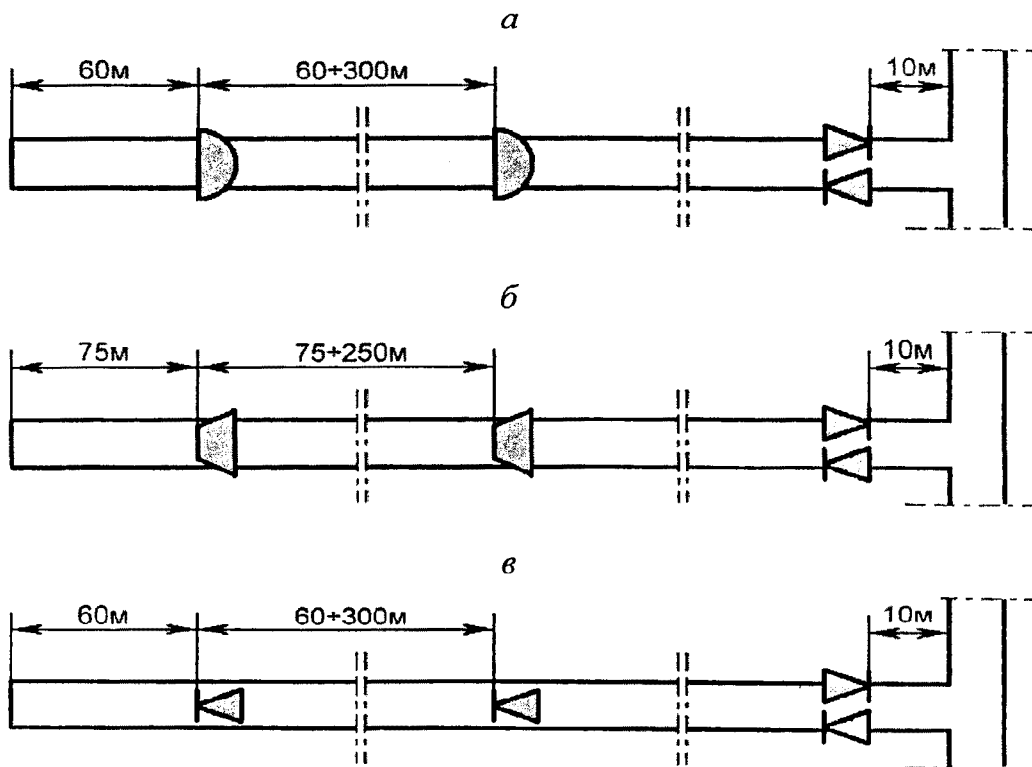
Рис. 3. Схемы установки заслонов в подготовительной выработке
