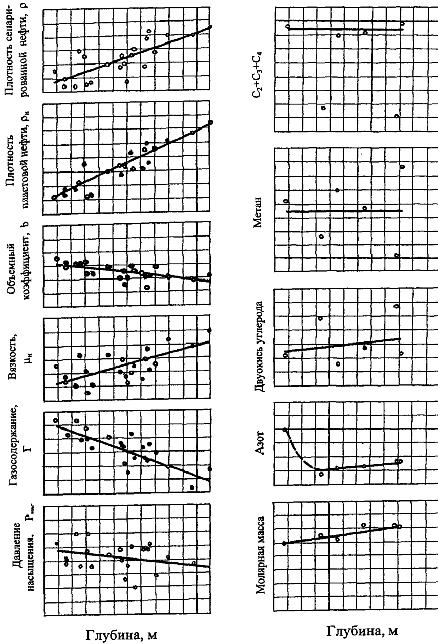
Рисунок 1- Вариант зависимости параметров пластовой нефти от глубины залегания пласта
