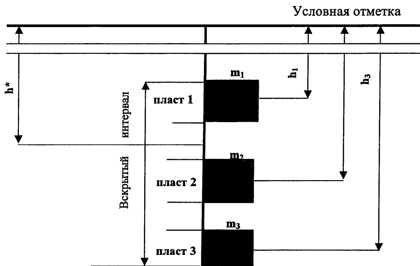
Рисунок 2- Вскрытые и работающие интервалы пласта
