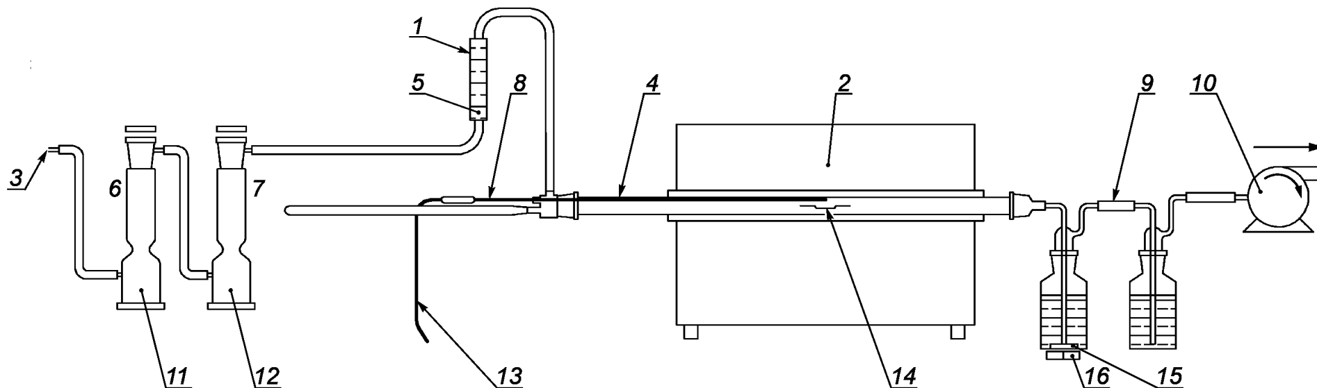
1 — ротаметр; 2 — печь; 3 — воздух окружающей среды; 4 — трубка из кварцевого стекла; 5 — игольчатый вентиль; 6 — активированный уголь; 7 — силикагель; 8 — термопара; 9 — промывочные сосуды; 10 — всасывающий насос; 11 — воздушный фильтр; 12 — осушитель воздуха; 13 — устройство для ввода лодочки для сжигания с испытуемым образцом; 14 — лодочка для сжигания с испытуемым образцом; 15 — стержень магнитной мешалки; 16 — магнитная мешалка
