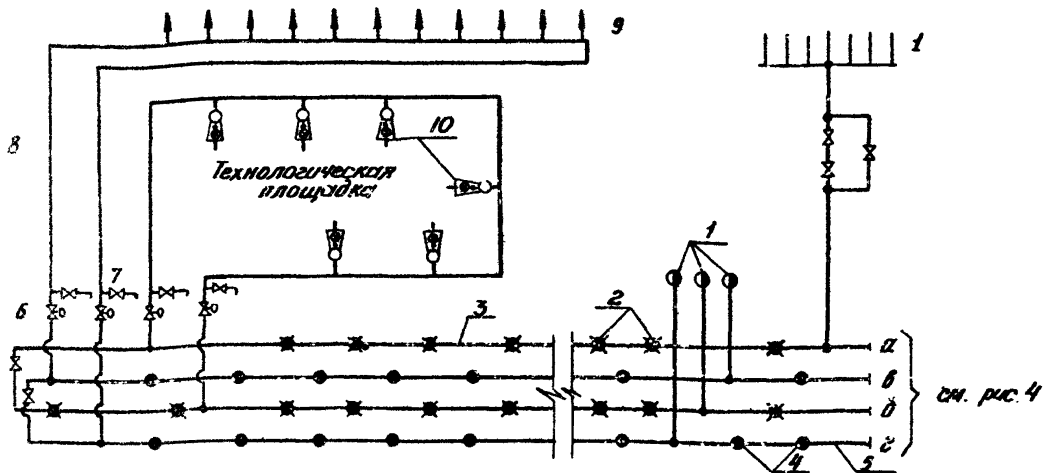
Рис. 1. Принципиальная схема СЯПЗ с водяной завесой.
