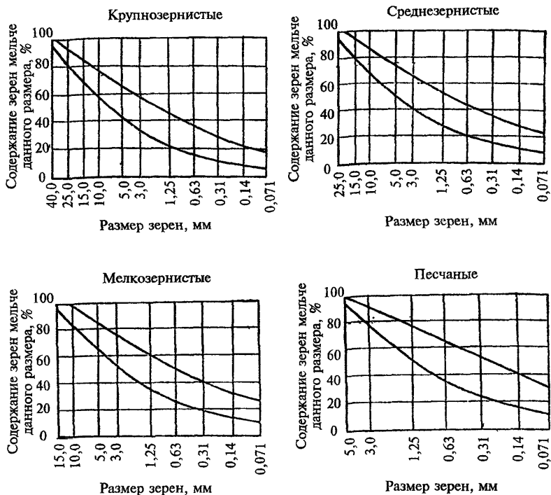
Рис. 1. Кривые зерновых составов плотных смесей непрерывной гранулометрии
