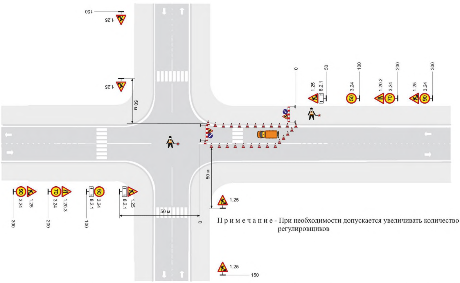
Рисунок Б.39 - Пересечение автомобильных дорог в одном уровне. Рабочая зона краткосрочных работ по нанесению дорожной разметки на полосу движения. Пропуск транспортных средств по полосе встречного движения с помощью регулировщиков
