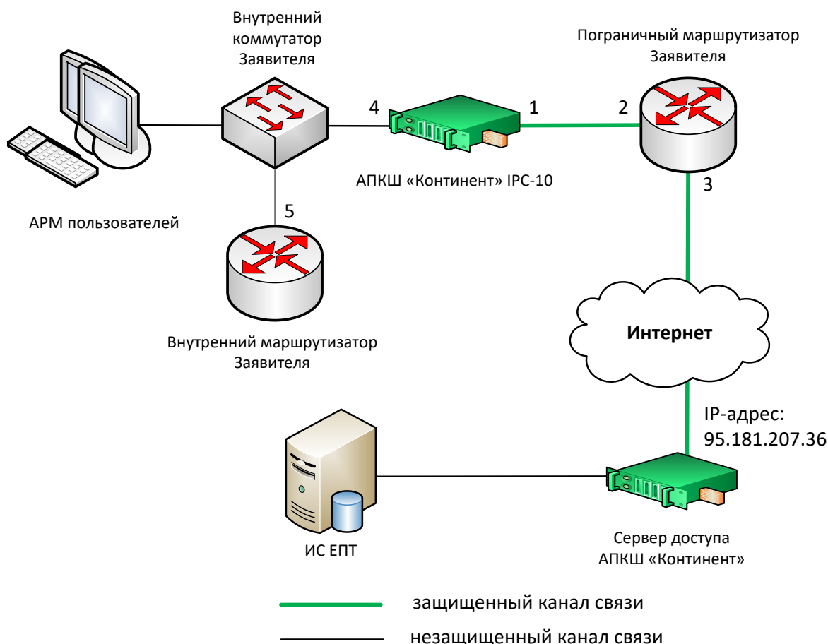
Рисунок 2. Схема подключения при использовании АПКШ «Континент» IPC-10
