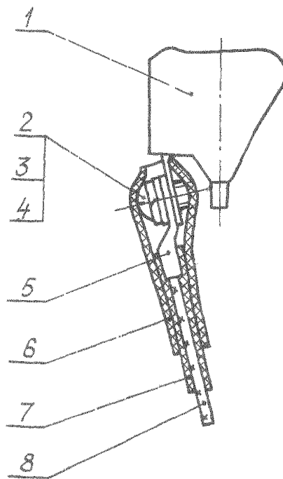
1 - электроэлемент; 2 - шайба защитная; 3 - шайба пружинная; 4 - винт; 5 - наконечник; 6,7 - трубка электроизоляционная термоусаживаемая; 8 - провод
