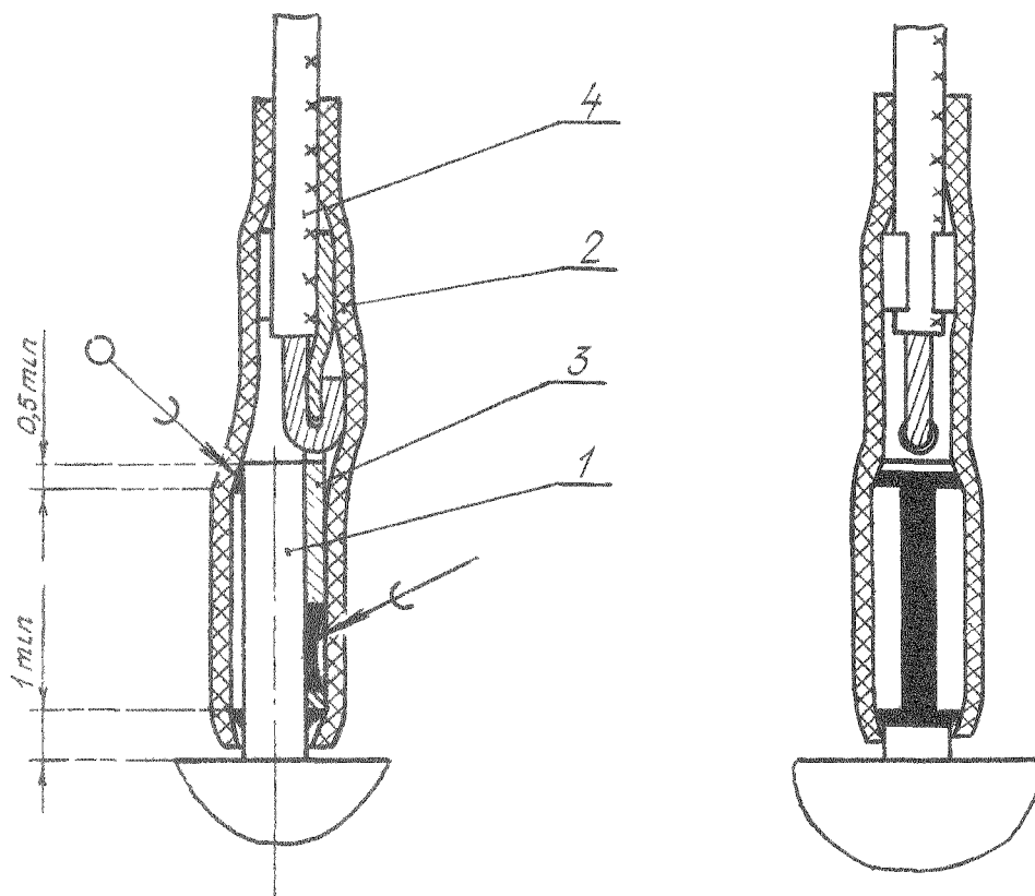
1 - контакт; 2 - трубка электроизоляционная; 3 - наконечник по ОСТ 1 13709-81; 4 - провод
