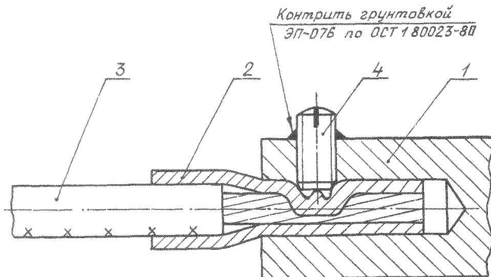
1 - электроэлемент; 2 - наконечник по ОСТ 1 13700-81; 3 - провод; 4 - винт Черт. 32
