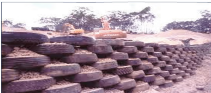
Рисунок 11.52 - Невысокая подпорная стенка шумозащитного вала из утилизированных автомобильных покрышек
