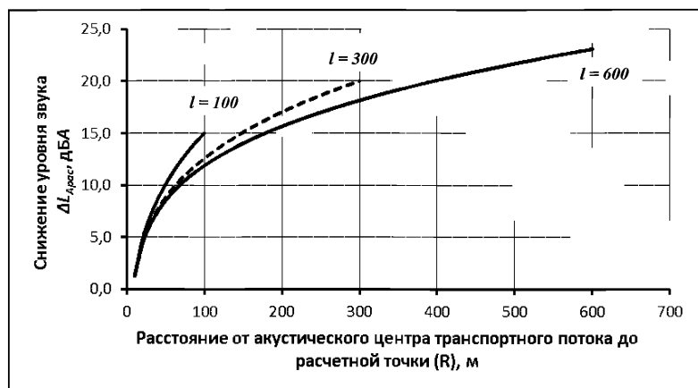
Рисунок Б.2 - Снижение уровня звука транспортного потока, в зависимости от увеличения расстояния до расчетной точки ( \Delta L_{Арас} ) при длинах подлежащих расчету участков дороги ( l ) 100 м, 300 м и 600 м
