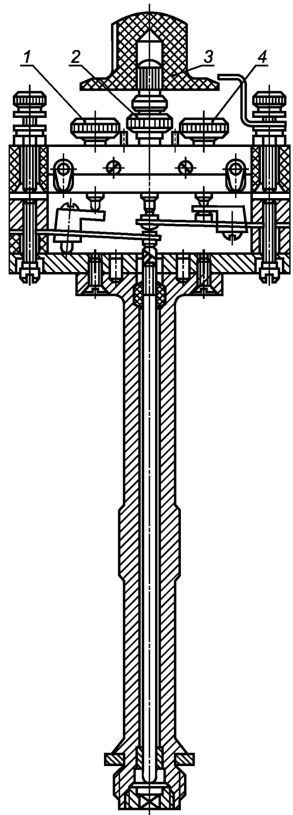
1, 4 — установочные винты; 2 — центральный винт; 3 — регулировочный винт
