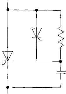
Рисунок А.1d — Пример гасящего контура Рисунок А.1 — Примеры форм сигнала и их контуров
