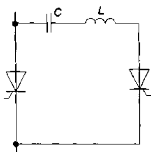
Рисунок А.1б — Пример контура коммутации
