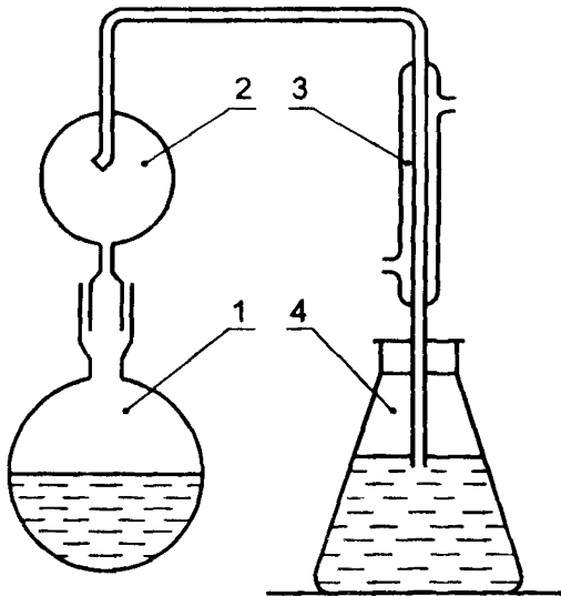
1 — круглодонная колба, 2 — каплеуловитель, 3 — холодильник, 4 — присная колба
