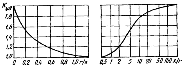
Кривые зависимости ударного коэффициента K_{уд} от отношений r/x и x/r
