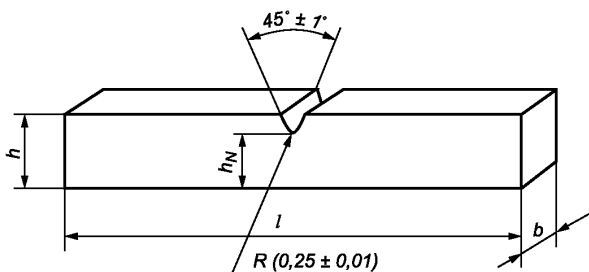
Рисунок 5 — Надрез типа В
