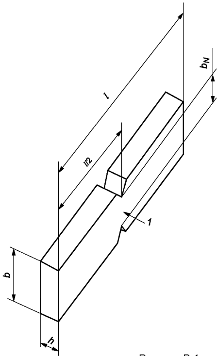
Рисунок В.1 — Образец с двойным V-образным надрезом
