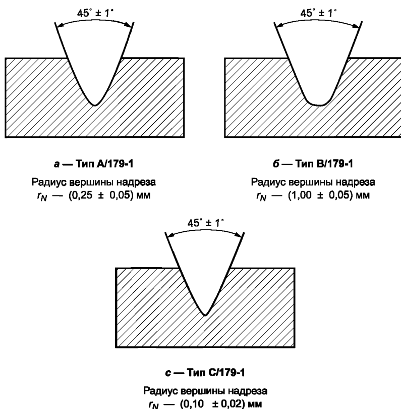
Рисунок 6 — Типы надрезов
