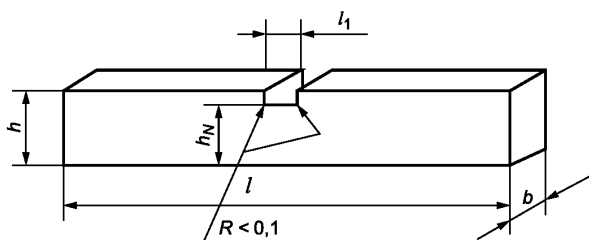
Рисунок 4 — Надрез типа А
