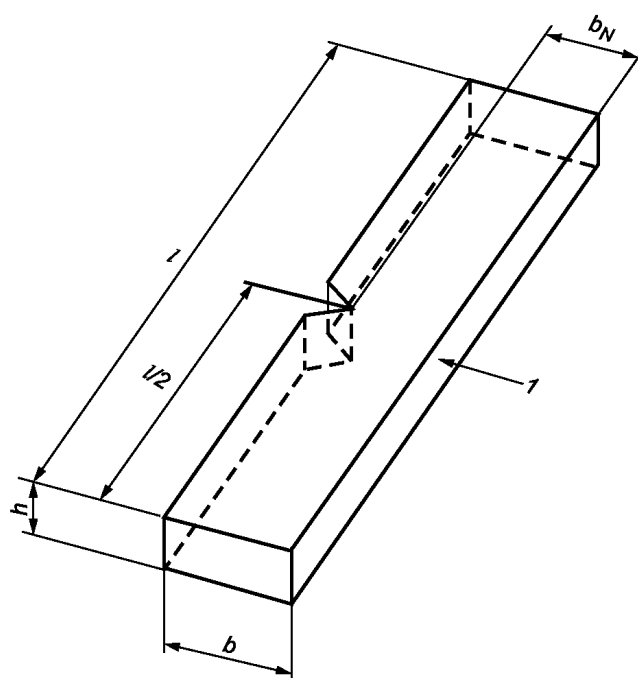
Рисунок 1 — Удар по Шарпи в ребро в образце с надрезом
