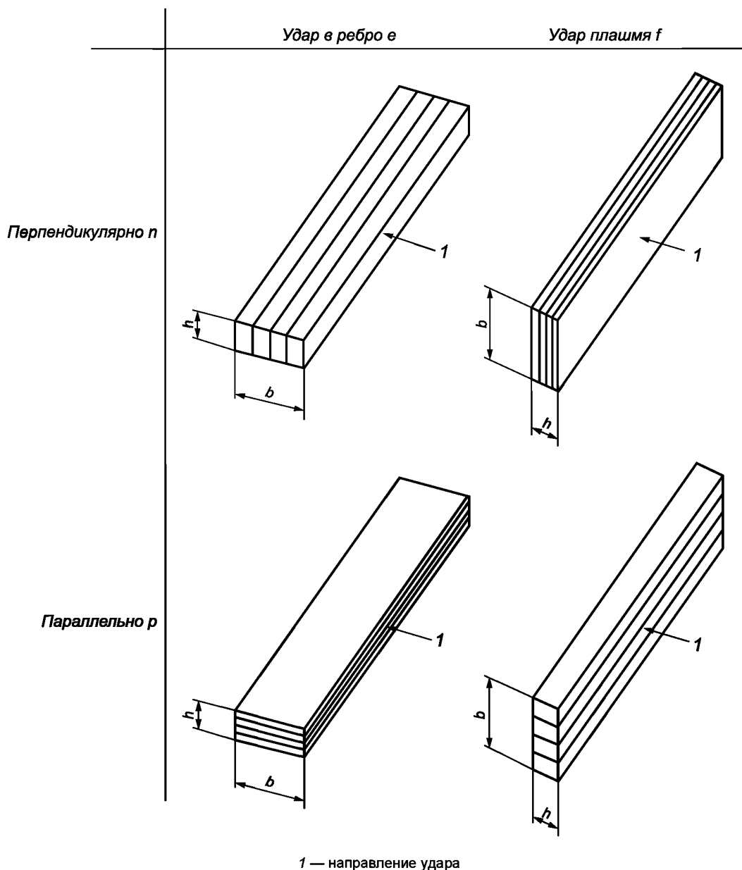
Рисунок 3 — Схема обозначений, описывающих направление удара
