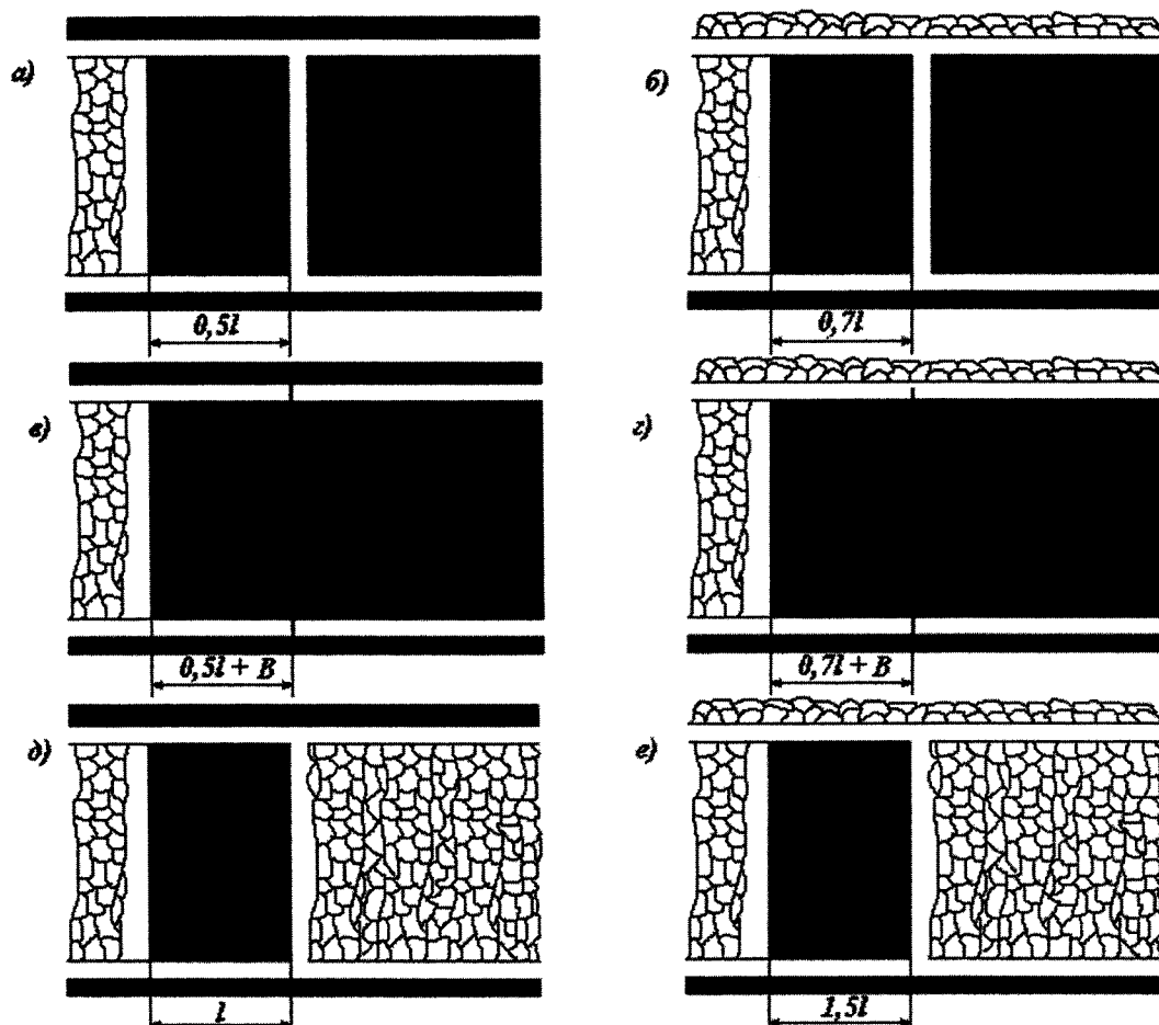
Рис. 1. Схемы определения d:
