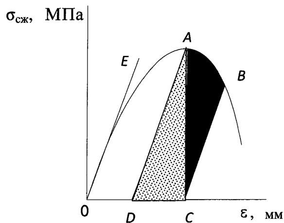
Рис. 2. График зависимости \sigma_{сж} от \epsilon
