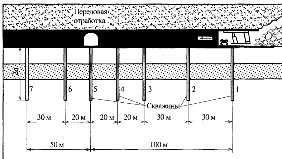
Рис. 1. Схема заложения геолого-разведочных скважин
