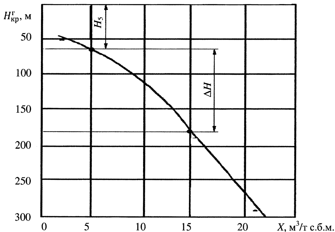
Рис. 3. Схема определения H_{кр}^r и grad X с использованием графика нарастания природной газоносности с глубиной
