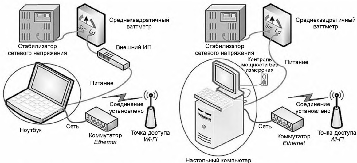
Рисунок 1 — Типичная испытательная установка
