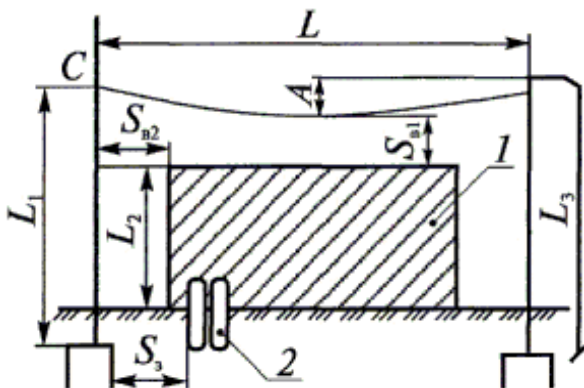
Рисунок 2. Отдельно стоящий тросовый молниеотвод: L - расстояние между молниеотводами; L_1 , L_3 - протяженность токопроводов; L_2 - высота защищаемого сооружения; S_{в1} , S_{в2} - наименьшие допустимые расстояния от тросового молниеотвода соответственно в точках А и С до защищаемого сооружения; S_з - наименьшее допустимое расстояние от заземления до металлических коммуникаций; 1 - защищаемое сооружение; 2 - металлические коммуникации.
