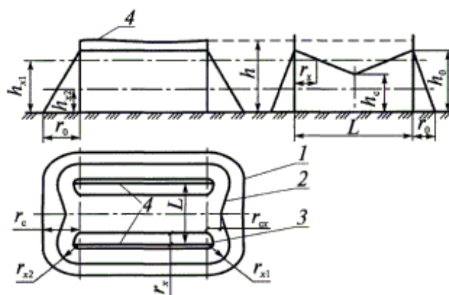
Рисунок 12. Схема зоны защиты двойного тросового молниеотвода:
