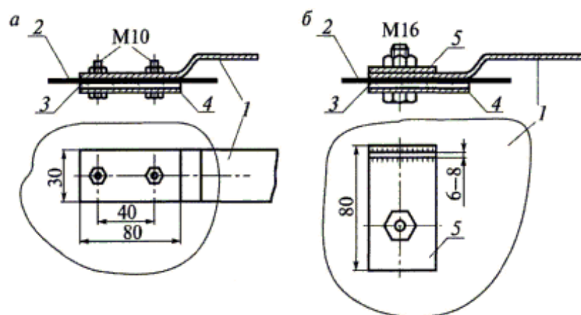
Рисунок 15. Зажим для присоединения плоского (а) и круглого (б) токоотводов к металлической кровле:
