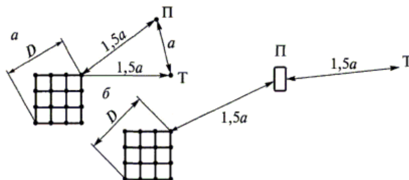
Рисунок 16. Двухлучевая (а) и однолучевая (б) схемы расположения электродов при измерении сопротивлений сложных заземлений и одиночных горизонтальных полос:
