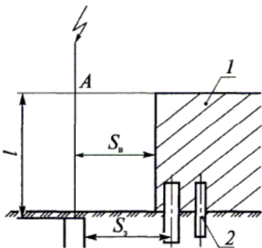
Рисунок 1. Отдельно стоящий стержневой молниеотвод: l - протяженность токопровода от точки А до заземлителя; S_{в} - наименьшее допустимое расстояние до защищаемого сооружения; S_{з} - наименьшее допустимое расстояние от заземлителя до металлических коммуникаций; 1 - защищаемое сооружение; 2 - металлические коммуникации
