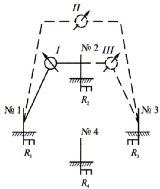
Рисунок 17. Схема измерения сопротивления заземлителей способом трех измерений
