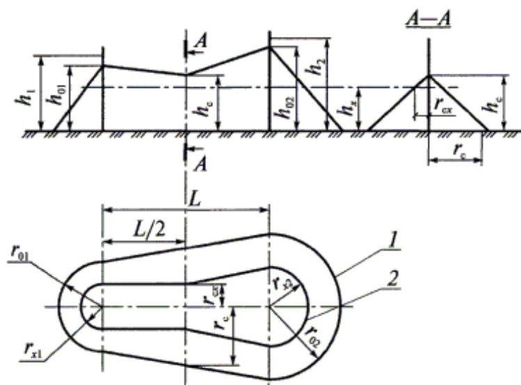
Рисунок 9. Схема зоны защиты двух стержневых молниеотводов разной высоты:
