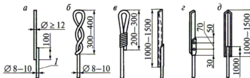
Рисунок 14. Конструкции молниеприемников из круглой стали (а), стальной проволоки диаметром 2 - 3 мм (б), стальной трубы (в), полосовой стали (г), угловой стали (д):
