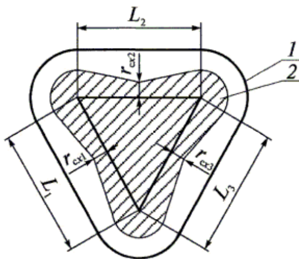
Рисунок 10. Схема зоны защиты (в плане) многократного стержневого молниеотвода:
