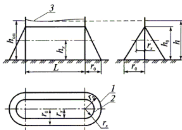
Рисунок 11. Схема зоны защиты одиночного тросового молниеотвода:
