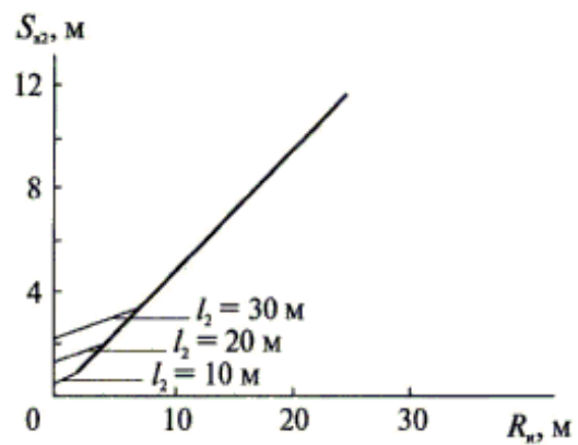
Рисунок 5. Наименьшие допустимые расстояния от молниеотвода до защищаемого
