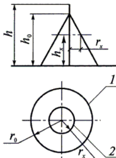
Рисунок 7. Схема зоны защиты одиночного стержневого молниеотвода:
