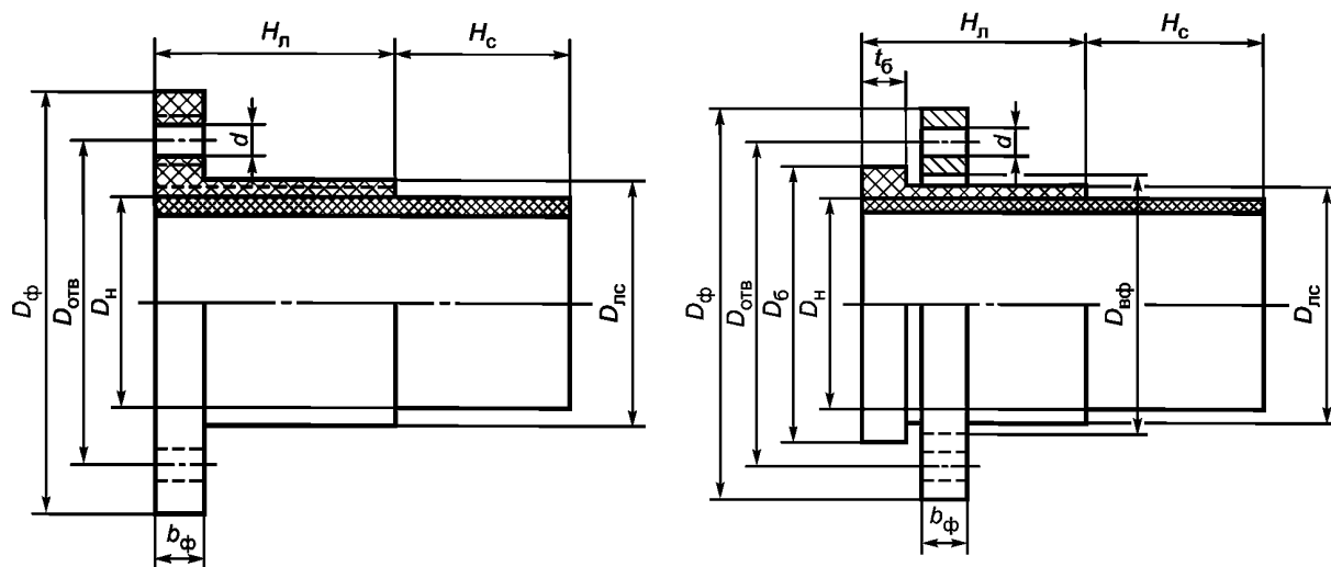
а — Фиксированный фланец
