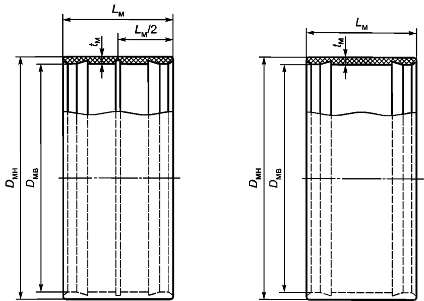
а – Муфта с центральным упором б – Муфта без центрального упора
