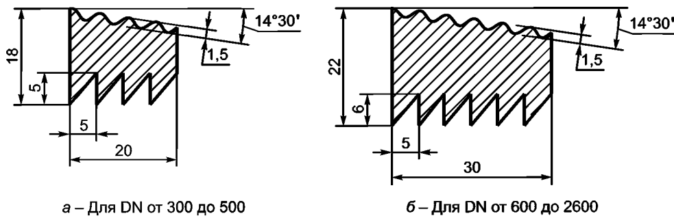
Рисунок Г.1 — Профили уплотнительных колец
