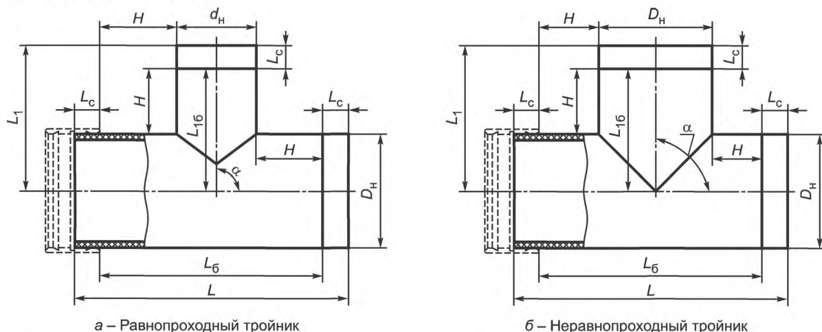
Рисунок 6 — Основные размеры тройников
