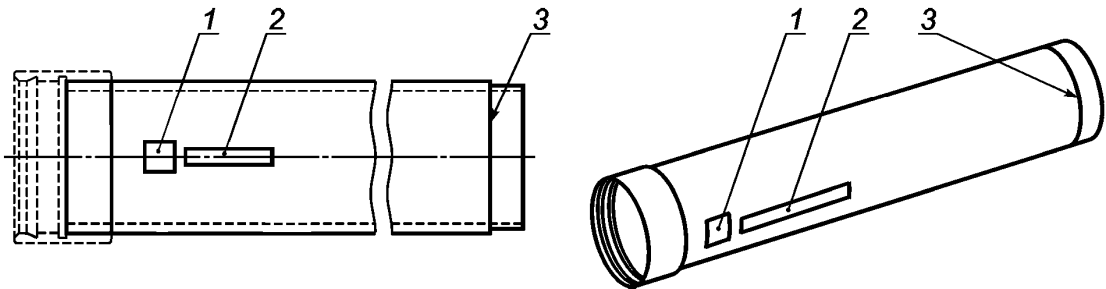
1 — место размещения ярлыка; 2 — место размещения условного обозначения; 3 — маркировочная линия на установочную муфту
