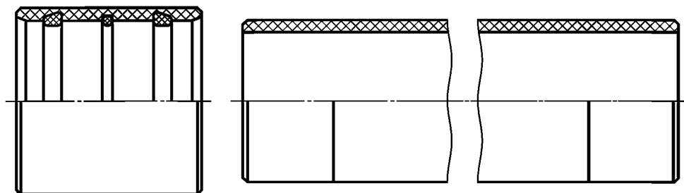
Рисунок 8 — Раздельная комплектация труб и муфт
