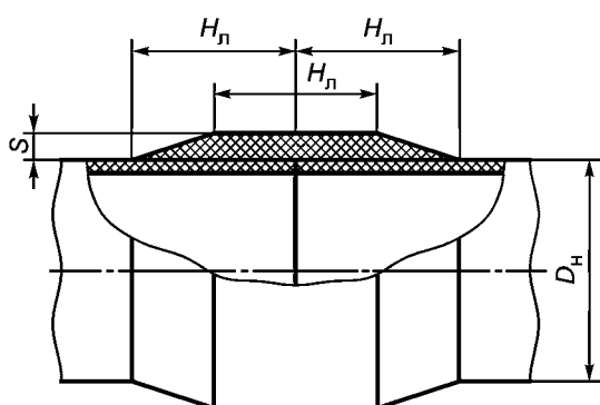
а — Общий вид соединения
