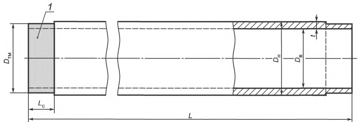
1 — калиброванная часть трубы для установки муфты; D_n — наружный диаметр; t — толщина стенки; L — длина трубы; D_{tm} — диаметр под муфтовое соединение (диаметр калиброванной части трубы); D_v — внутренний диаметр; L_c — длина соединения (длина калиброванной части трубы под муфтовое соединение)
