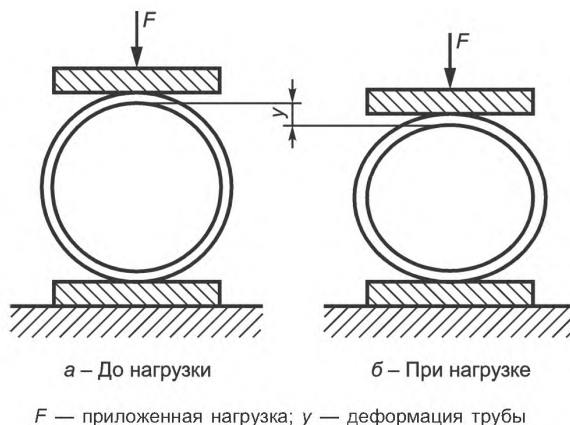
Рисунок 10 — Схема испытания на нагрузочной машине
