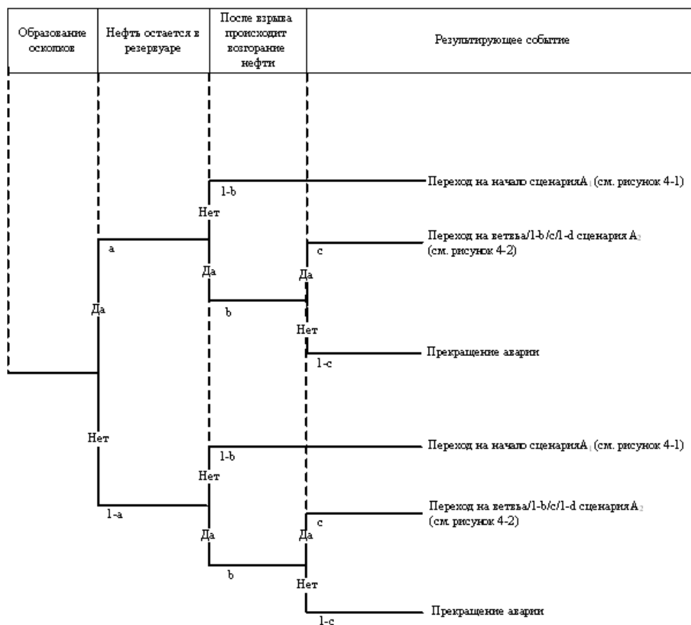
Рис. 3 "Дерево событий" при взрыве внутри наземного резервуара (сценарий А 3 )
