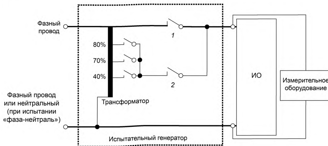
1, 2 — попеременно коммутируемые переключатели
