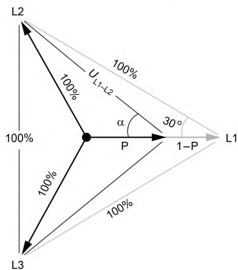
Рисунок С.1 — Векторы напряжений при провале напряжения «фаза—нейтраль»
