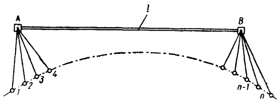
Рис. 3. Схема съёмки кривой с базиса: 1, 2 ... n —точки на оси пути; — · — · — ось пути
