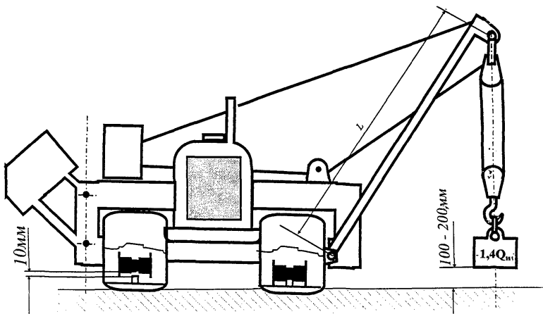
Рис.1 Схема нагружения крана-трубоукладчика
