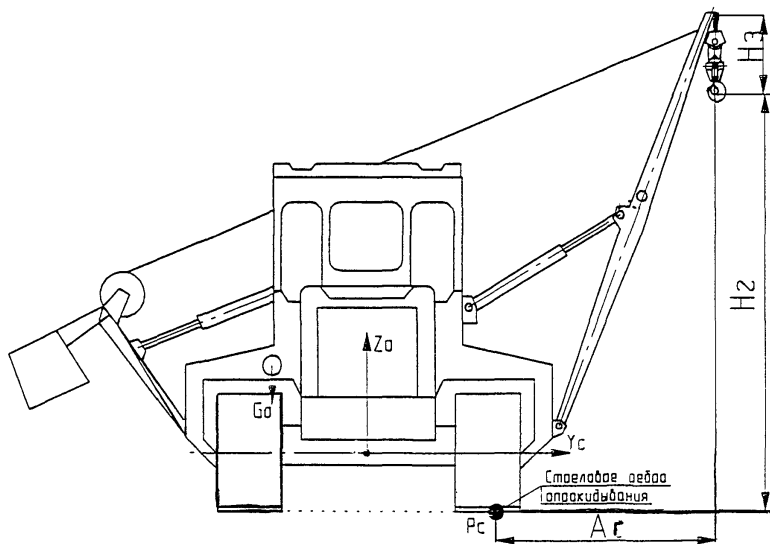
Рис.2 К определению вылета крана-трубоукладчика
