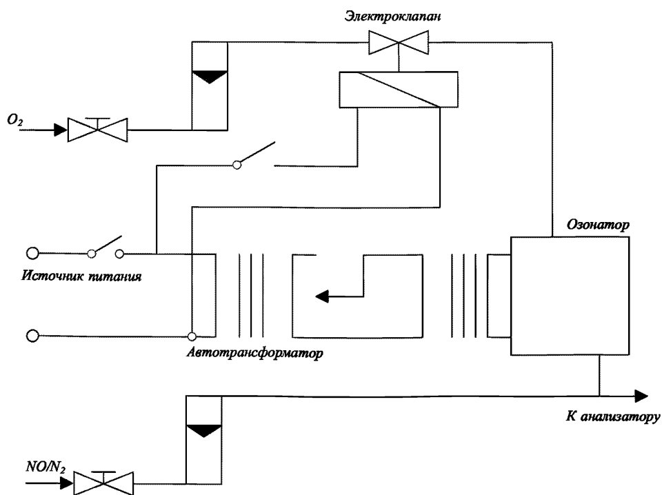
Рис. 11.1 Схема установки для определения КПД конвертера
