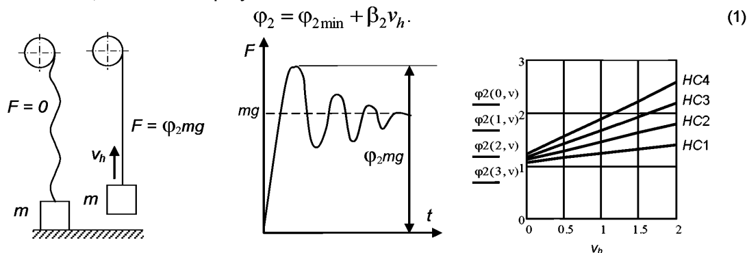
Рисунок 1 – Схемы к определению коэффициента \Phi_2
