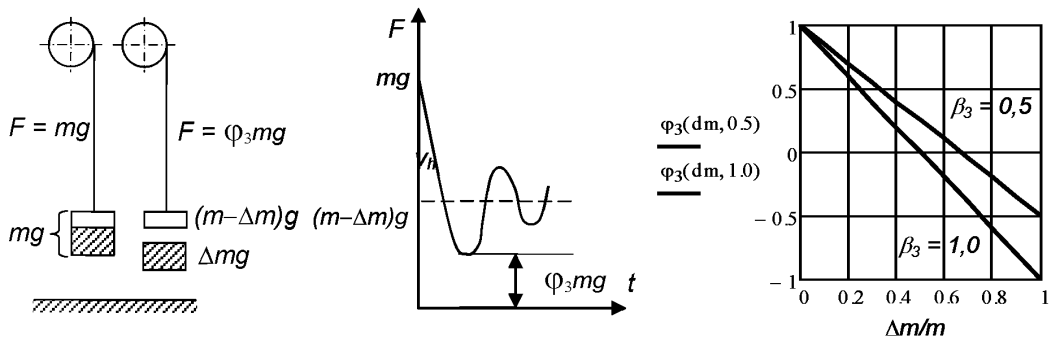
Рисунок 2 – Схемы к определению коэффициента \varphi_3
