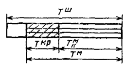
Черт. 2. Хронограммы штучного времени
