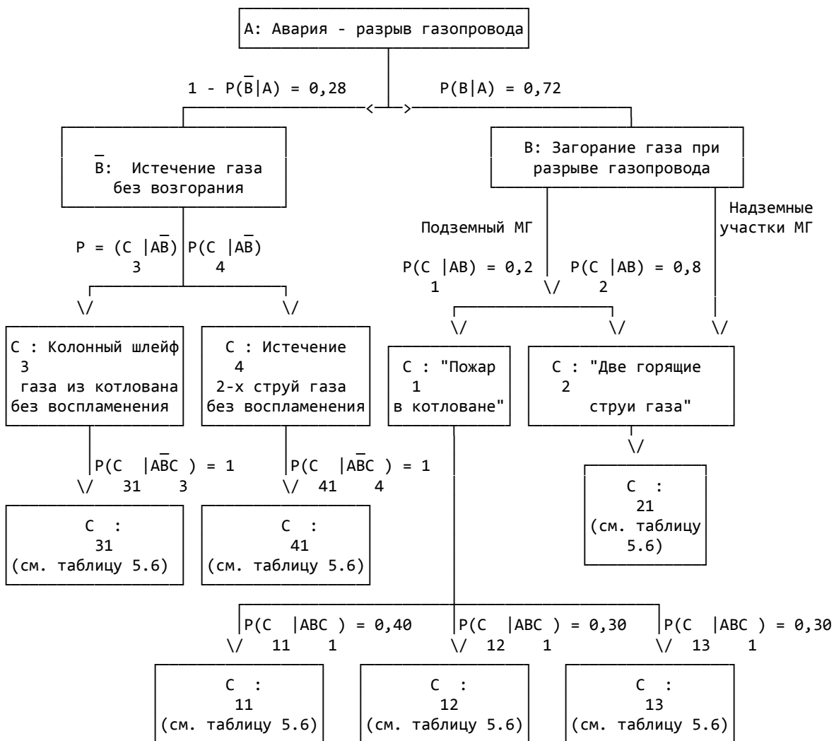
Рисунок 5.1. Упрощенное дерево событий для идентификации
