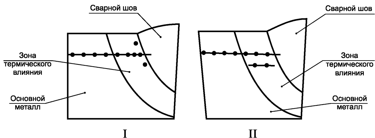
Схемы замеров твердости: I — основная, II — дополнительная
