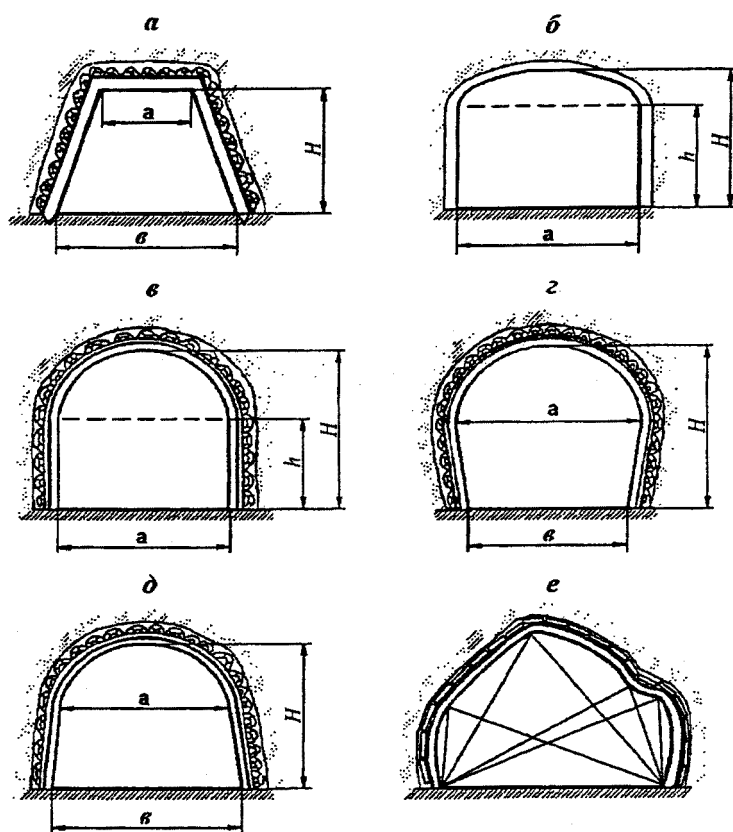
Рис. 2. Определение площадей поперечного сечения
