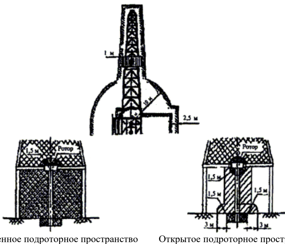
Рис. 2. Буровая установка с укрытием и привышечным сооружением для бурения скважин на море и месторождениях, содержащих сернистый водород
