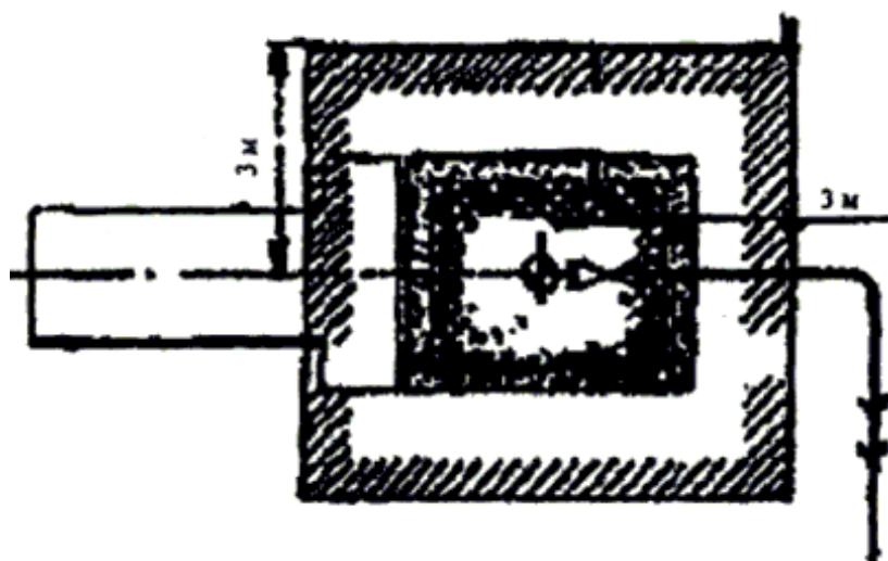
Рис. 5. Открытые пространства вокруг фонтанных арматур
