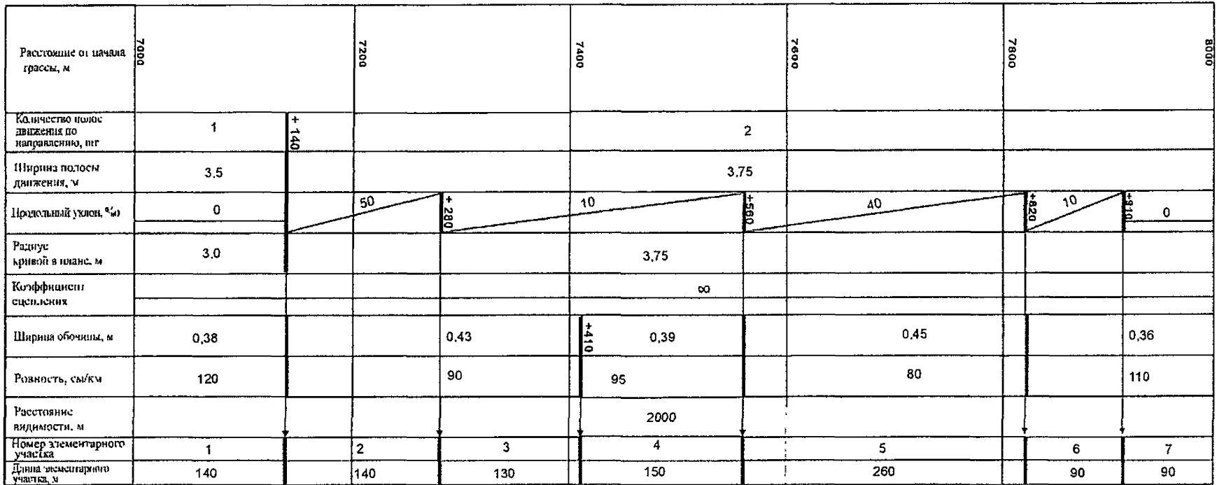
Рисунок В.2 – Типовая форма участка дороги после проведения 1-го варианта ремонта (вариант 1)
