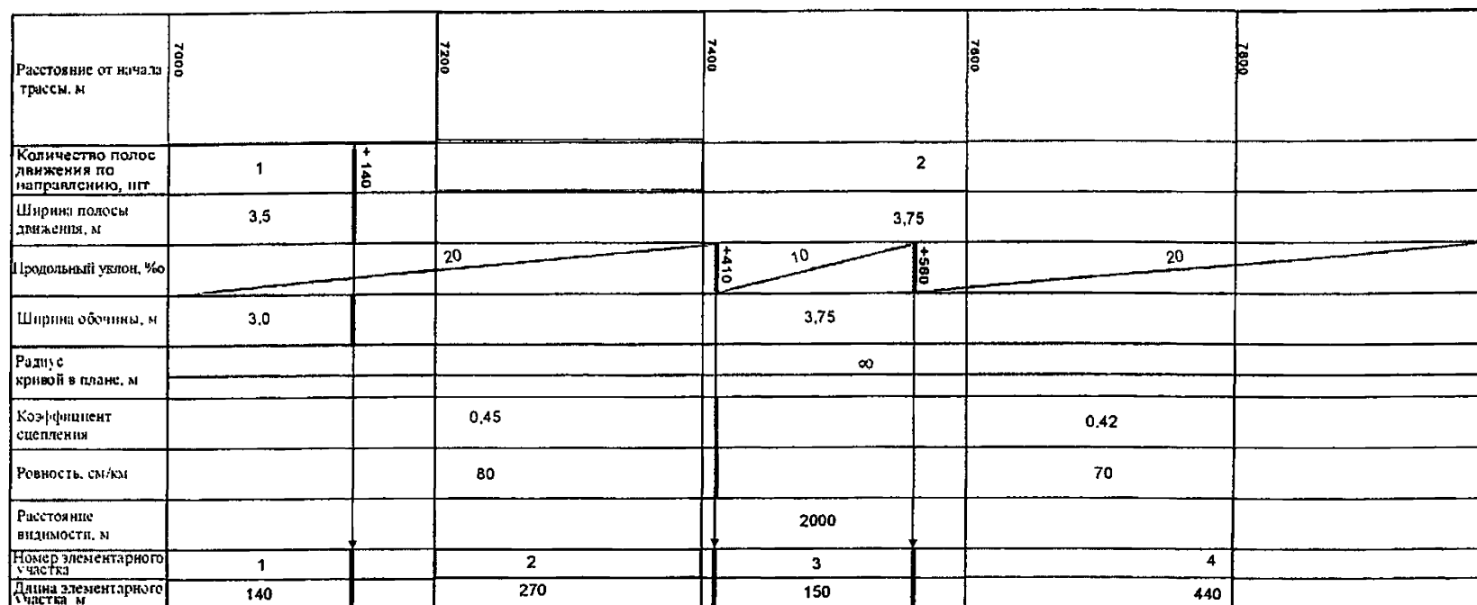
Рисунок В.4 – Типовая форма участка дороги после проведения 3-го варианта ремонта (вариант 3)
