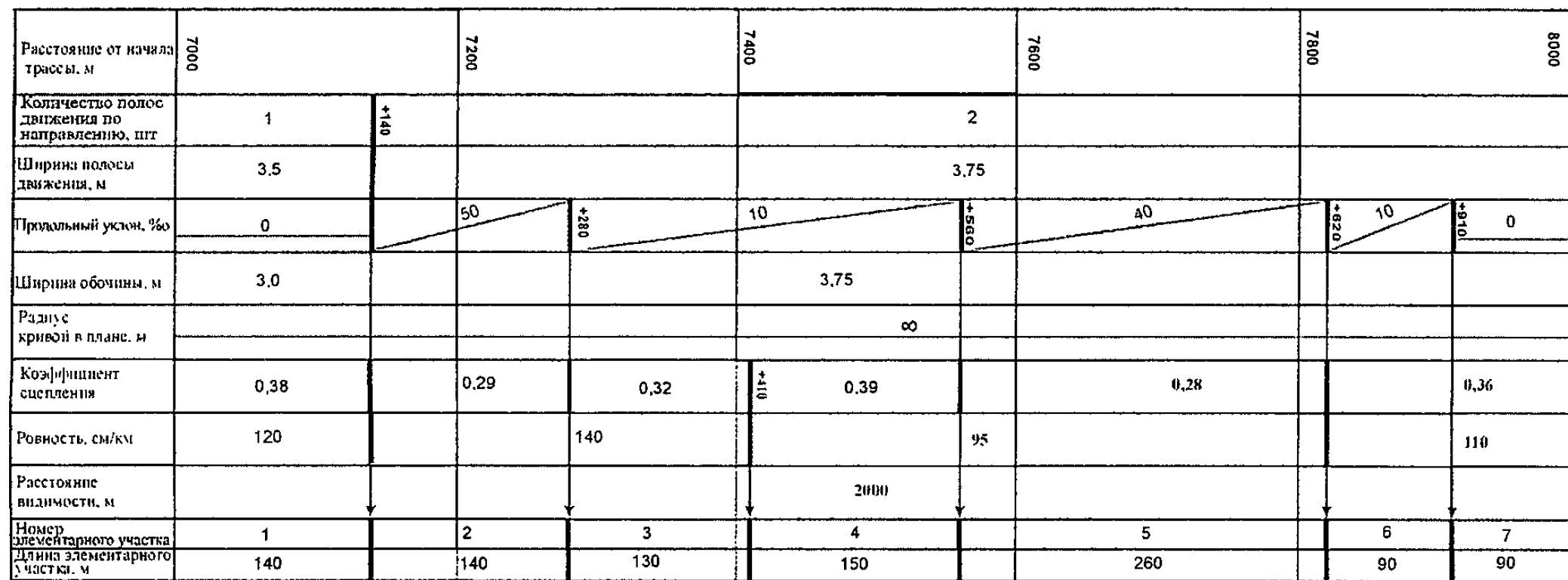
Рисунок В.1 – Типовая форма участка дороги (вариант 0)
