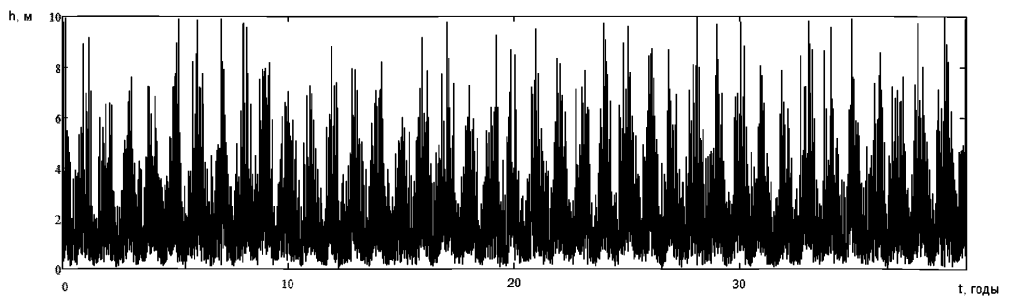
Рис. 4.1.2-1 Последовательность значительных высот волн для каждого синоптического срока (через 3 ч) за 40 лет
