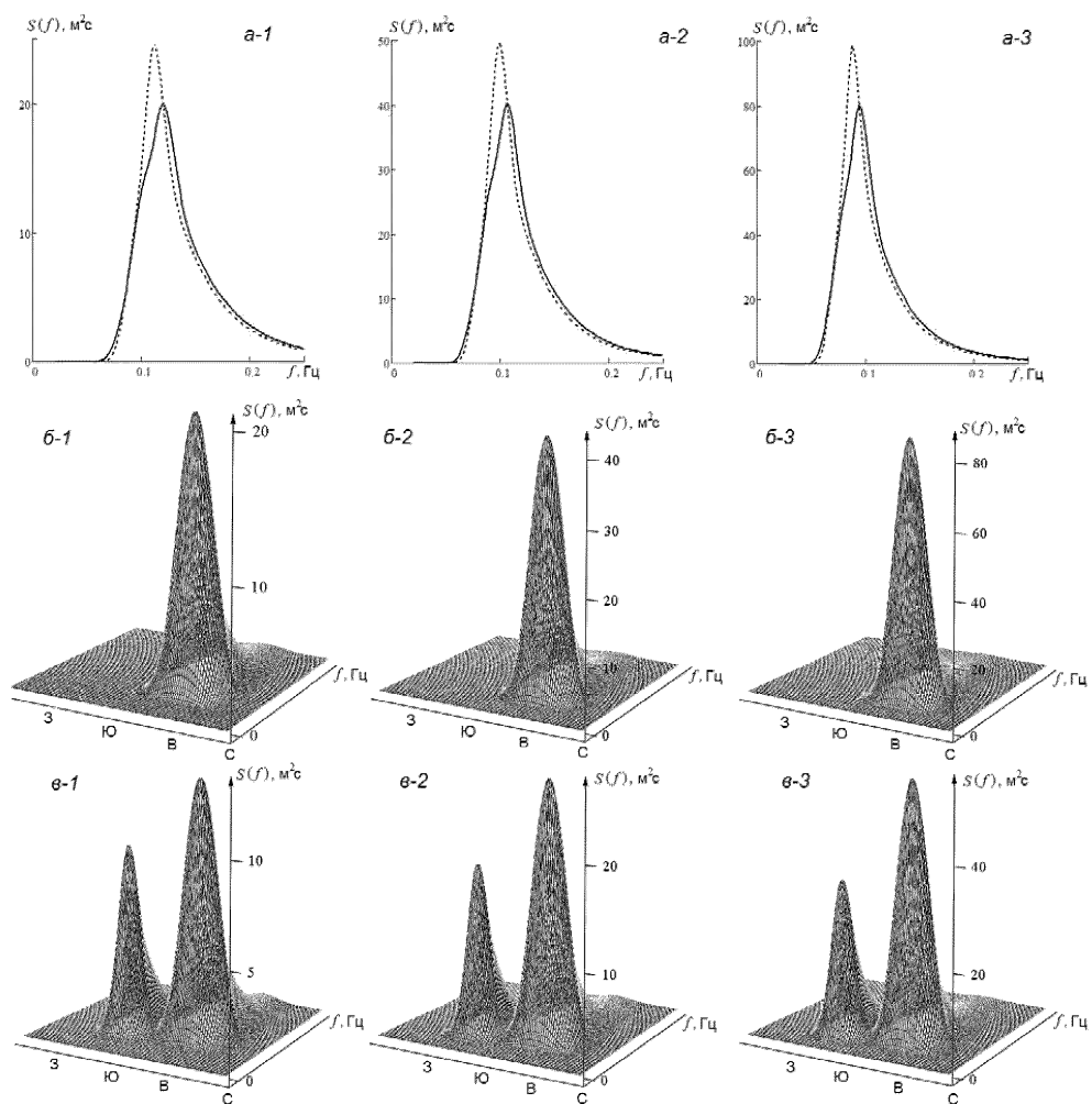
Рис. К.11 Климатические спектры экстремального волнения в Карском море: a – частотные спектры для классов I (пунктир) и IV (сплошная линия); б – частотно-направленный спектр для класса I; в – частотно-направленный спектр для класса IV; 1 – 1 раз в год; 2 – 1 раз в 10 лет; 3 – 1 раз в 100 лет
