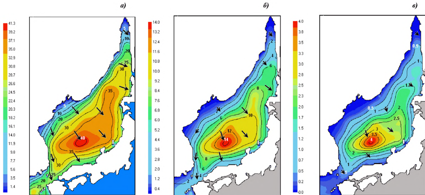
Рис. Я.9 Обеспеченность, %, высот волн (3 %-ной обеспеченности): a – более 2 м; б – более 4 м; в – более 6 м
