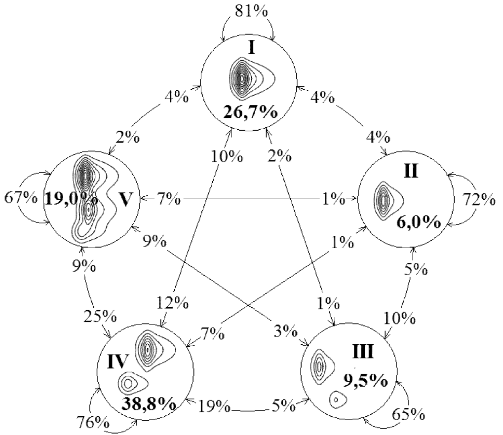
Рис. Я.10 «Звезда» климатических спектров. Японское море
