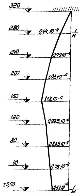
Рис.7. Эюра кривизны оси ствола трубы (3-е приближение)
