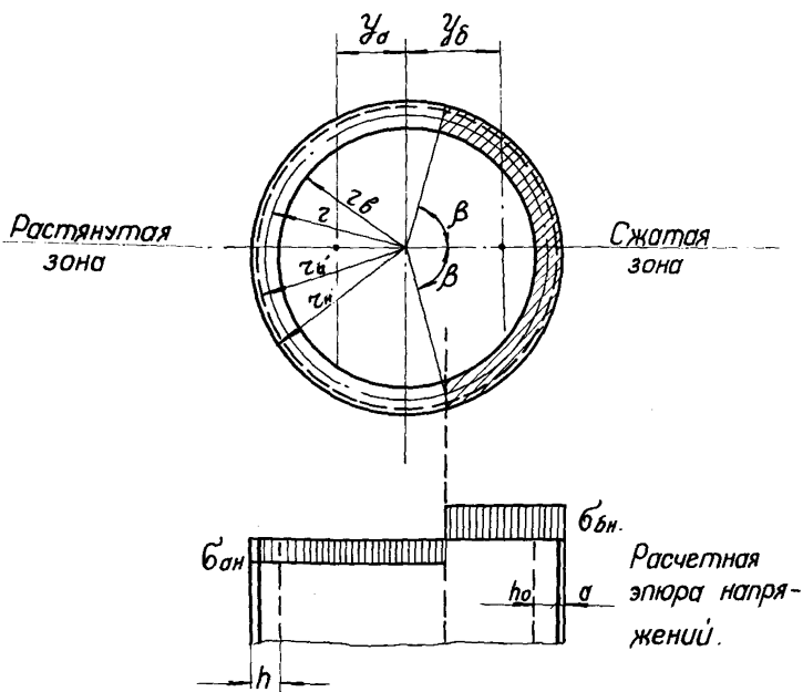
Рис. I. Расчетная схема горизонтального сечения труб и эпюра напряжений
