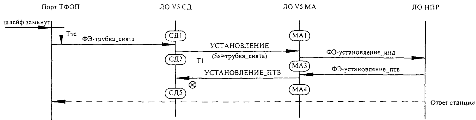
Рисунок Б.1 - Передача сообщений и ФЭ при занятии со стороны абонента А
