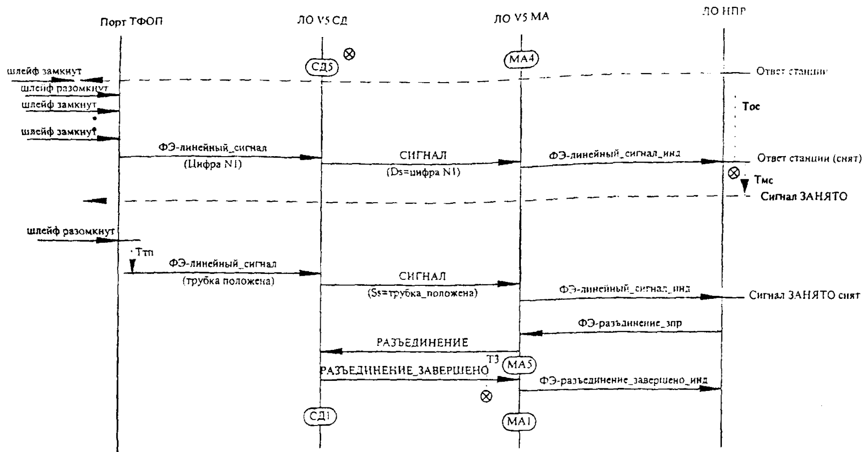
Рисунок Б.4 - Передача сообщений и ФЭ в случае превышения допустимого межсерийного интервала при наборе цифры
