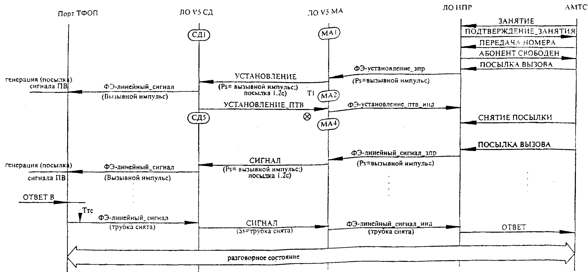
Рисунок Б.16 - Передача сообщений и ФЭ при входящем вызове от АМТС
