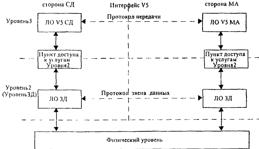
Рисунок 2 - Взаимодействие ЛО Уровня2 и ЛОВ5
