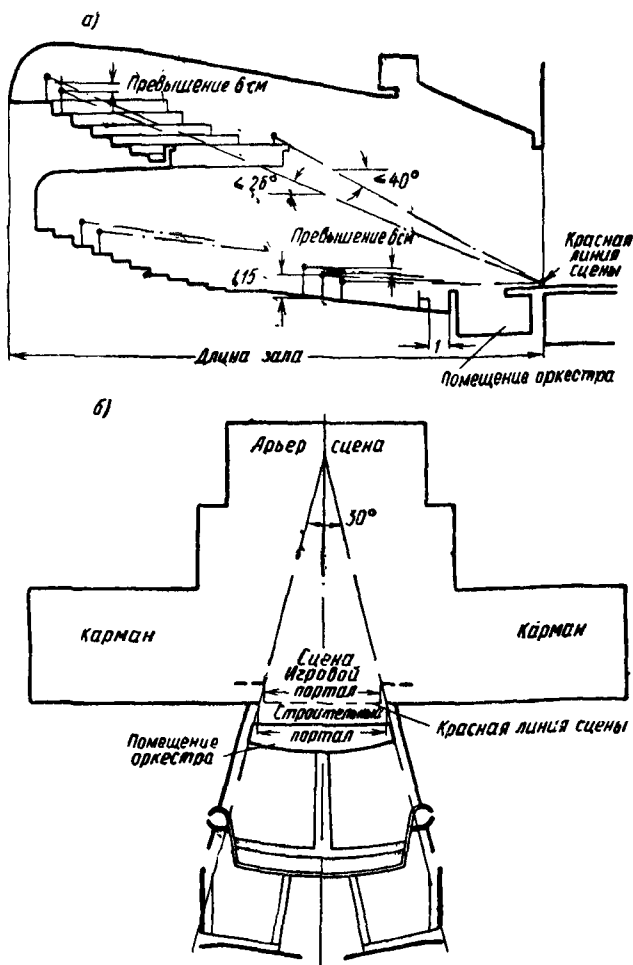
Рис. 1. Расчетные параметры зрительного зала театров с колосниковой сценой а—разрез зрительного зала; б—план зала и сцены
