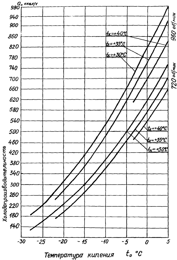
График холодопроизводительности компрессора АУУ-400
