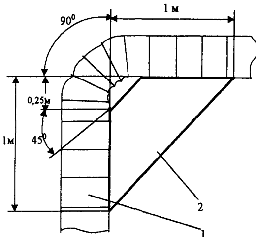
Рисунок 6. Шаблон для проверки угла сгиба всасывающего рукава:
