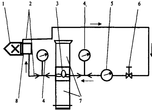
Рисунок 5. Схема размещения оборудования при проверке аэродинамических характеристик дымососа с гидротурбиной:
