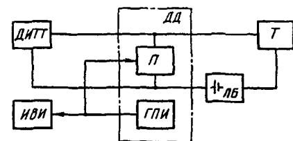
Схема измерения при дроблении бестоковой значащей посылки
