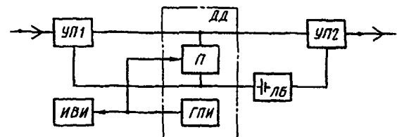
Схема измерения при дроблении минусовой значащей посылки
