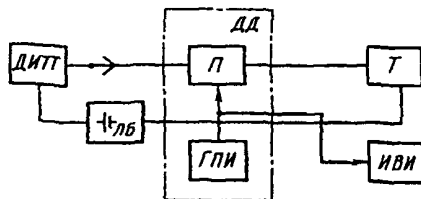
Схема измерения при дроблении токовой значащей посылки
