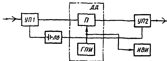
Схема измерения при дроблении плюсовой значащей посылки
