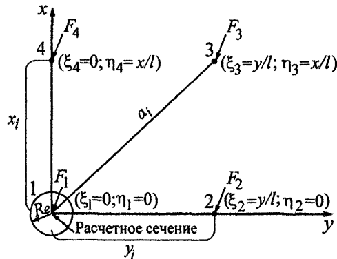
Рисунок 7.2 – Расчетная схема параметров загрузки опор воздушного судна
