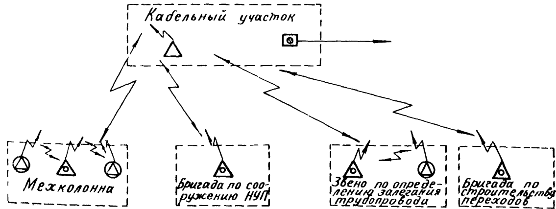
Рис.2. Схема организации радиосвязи кабельного участка: △ - радиостанция начальника кабельного участка; △ - мобильные УКВ радиостанции; ⊙ - портативные УКВ радиостанции; ⊠ - телефонный аппарат для выхода на сеть магистральной связи
