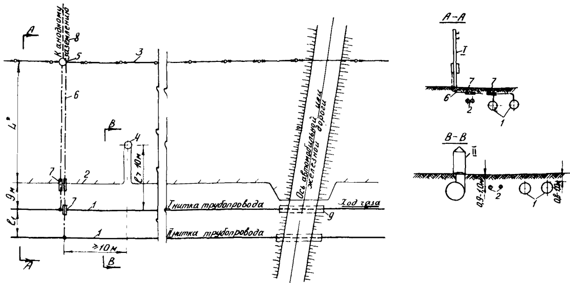
Рис.1. План размещения кабельных линий технологической связи вдоль действующих трубопроводов:
